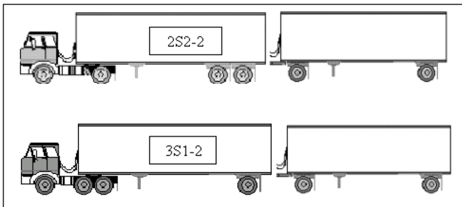
Figure 16:Klasi 12 — Kamiona Gjashtë Aksial Shumë Rimorkio
