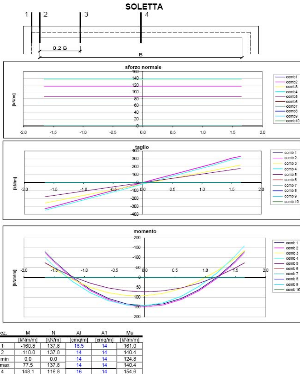
Fig.1.4 ( Diagrama e M,N,Q per Soleten + verifikimi SLU)
