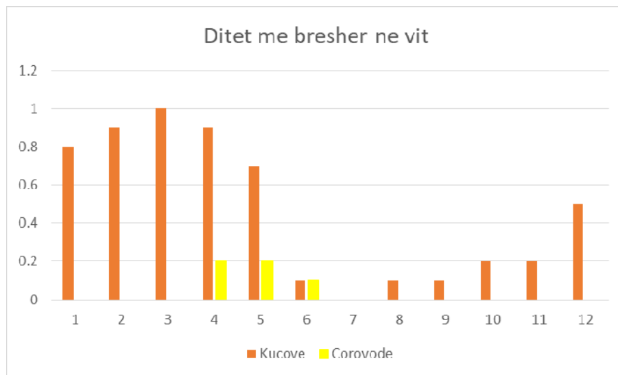
Figura: 0-7 Shperndarja vjetore e diteve me bresher
