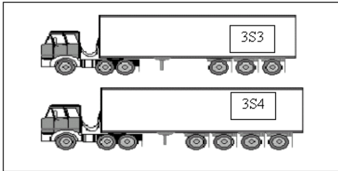
Figure 14:Klasi 10 — Kamiona Gjashtë ose Më Shumë Akse Një Rimorkio
