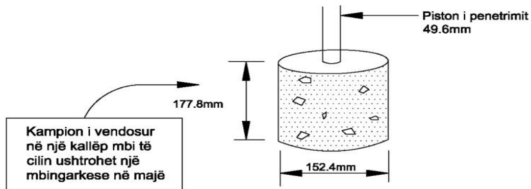
Figure 2:Kampioni tipik për CBR
