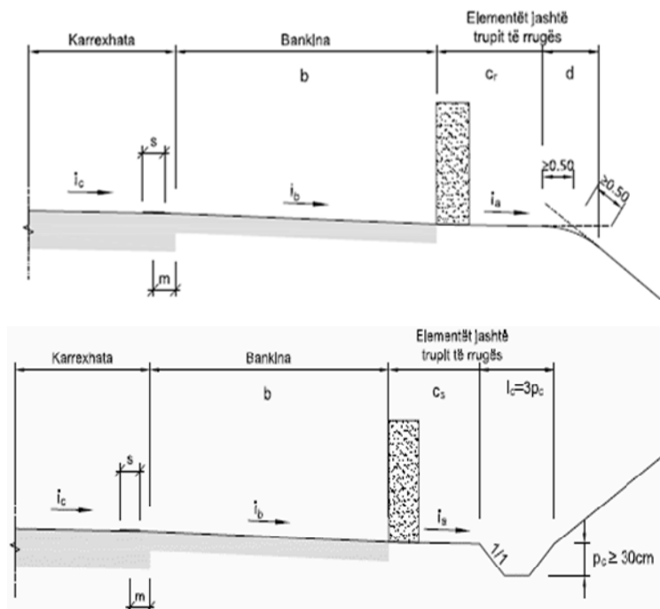
FIGURE 22- raste të ndryshme të dimensioneve të bankinës së paveshur
