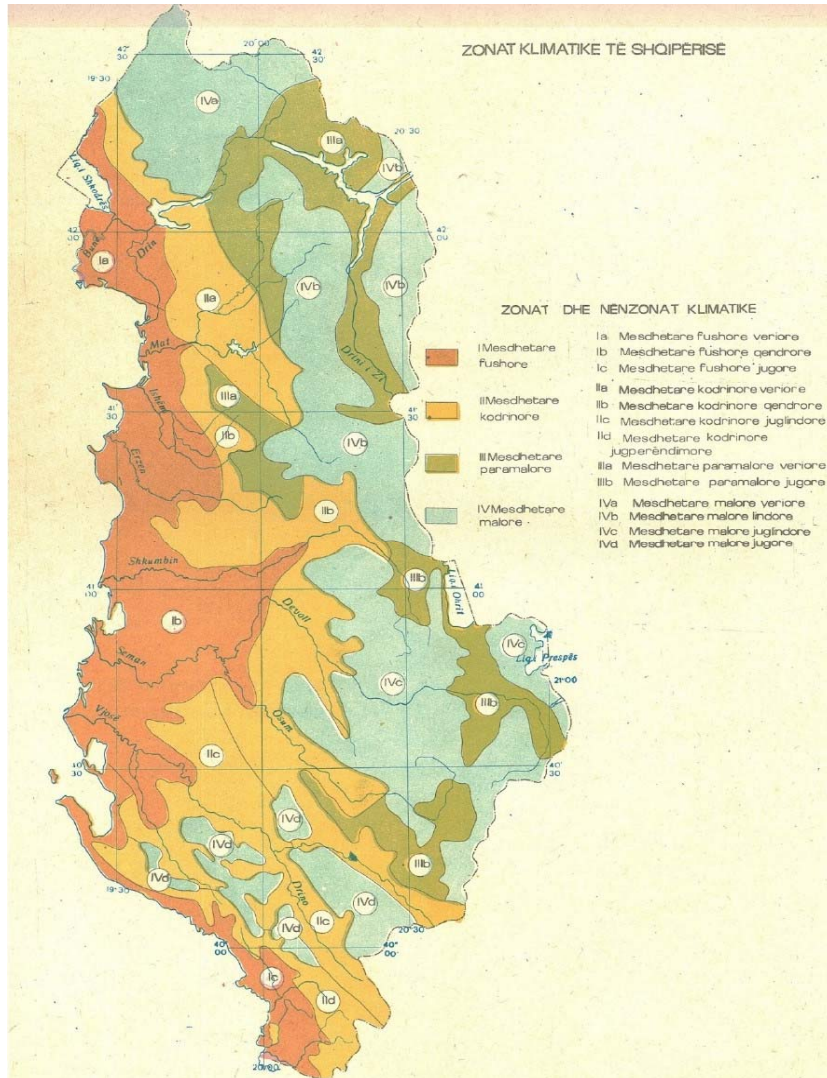
Fig. 2.2 Zonat klimatike te Shqiperise
