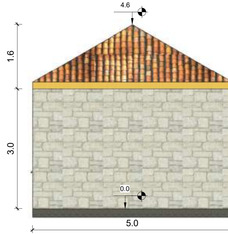
PRERJA 3-3
