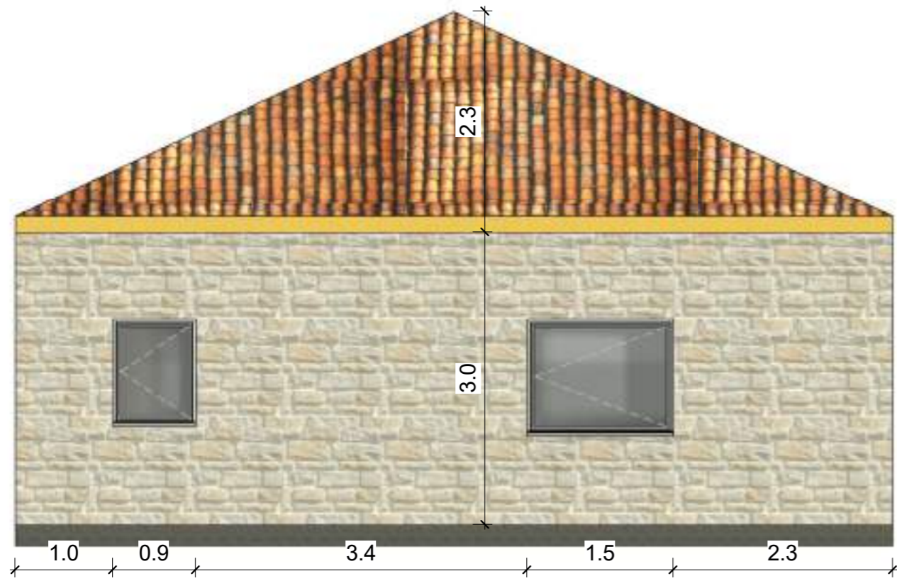
PRERJA 3-3
