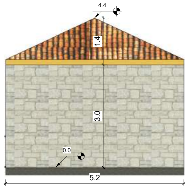
PRERJA 2-2
