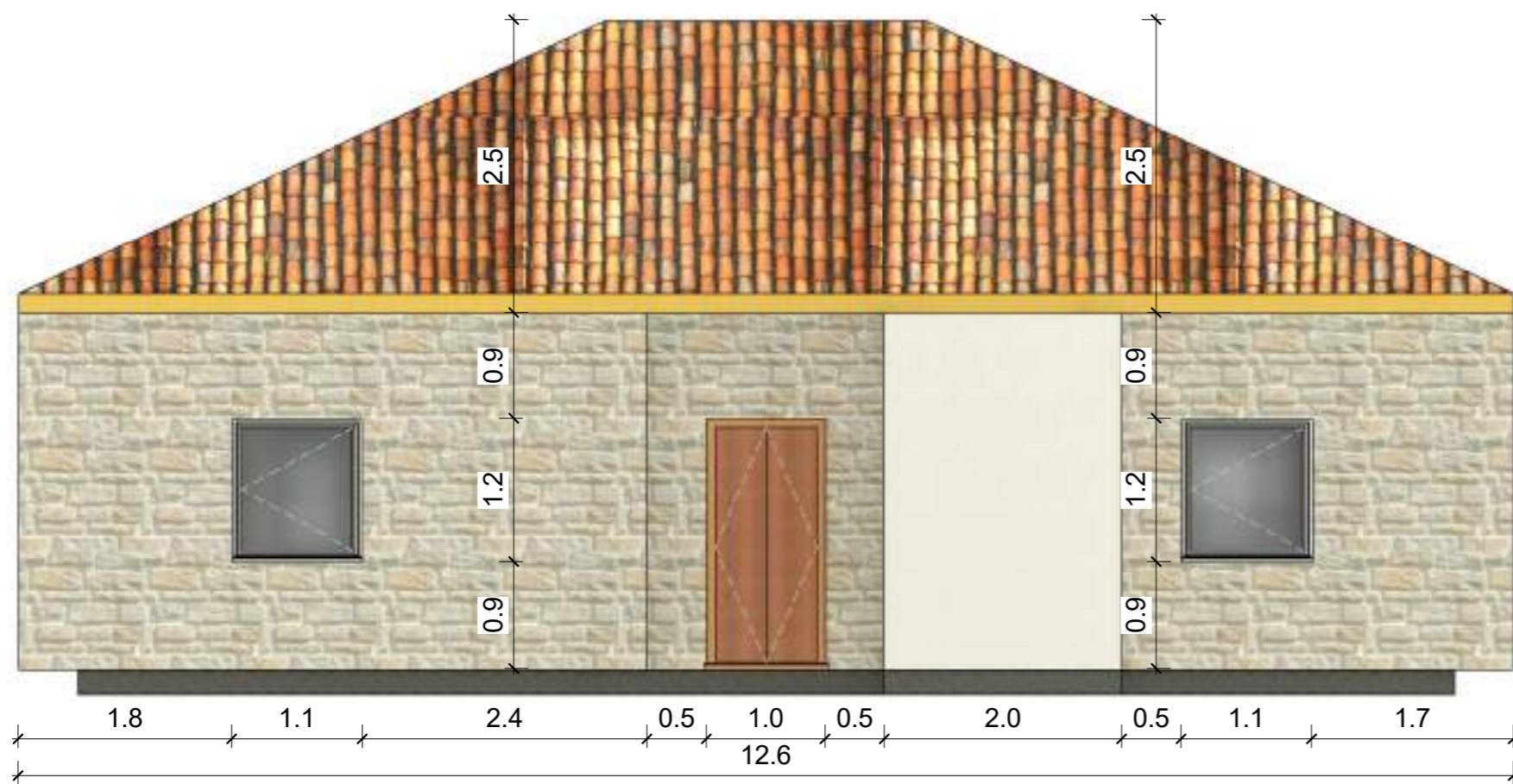
PRERJA 1-1
