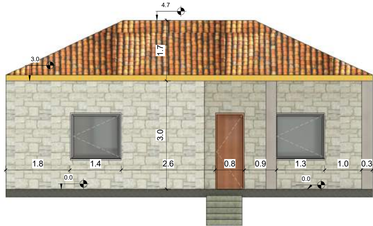
PRERJA 2-2
