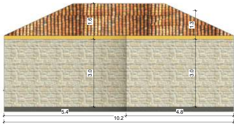
PRERJA 3-3
