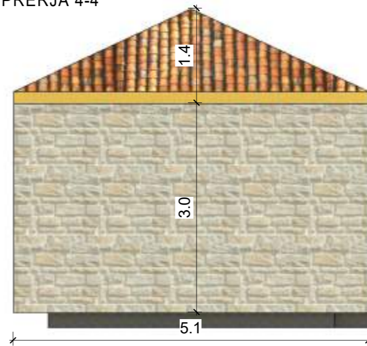
PRERJA 4-4
