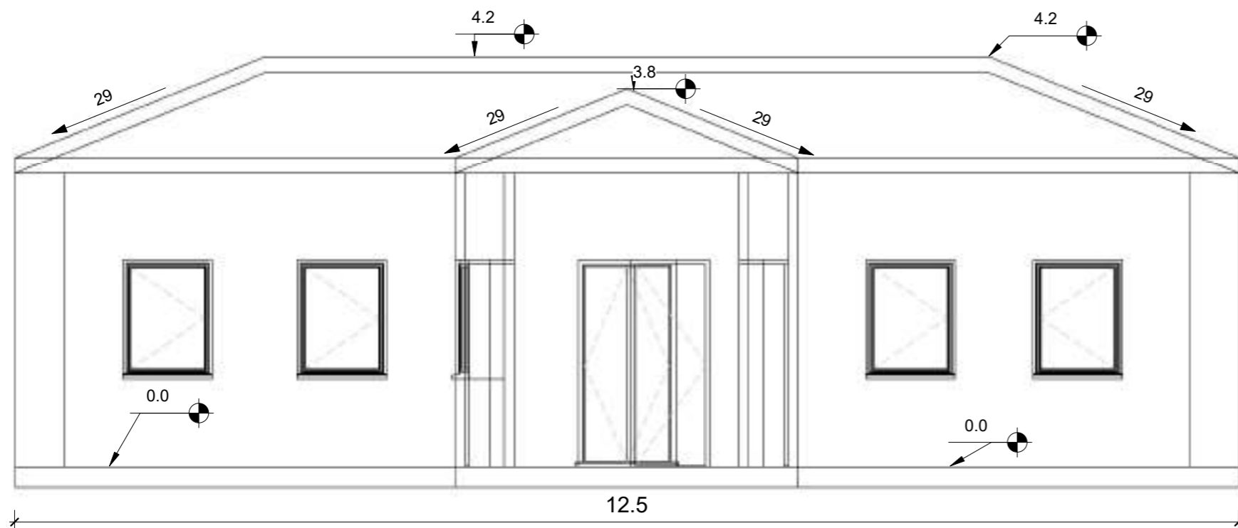
PRERJA 3-3
