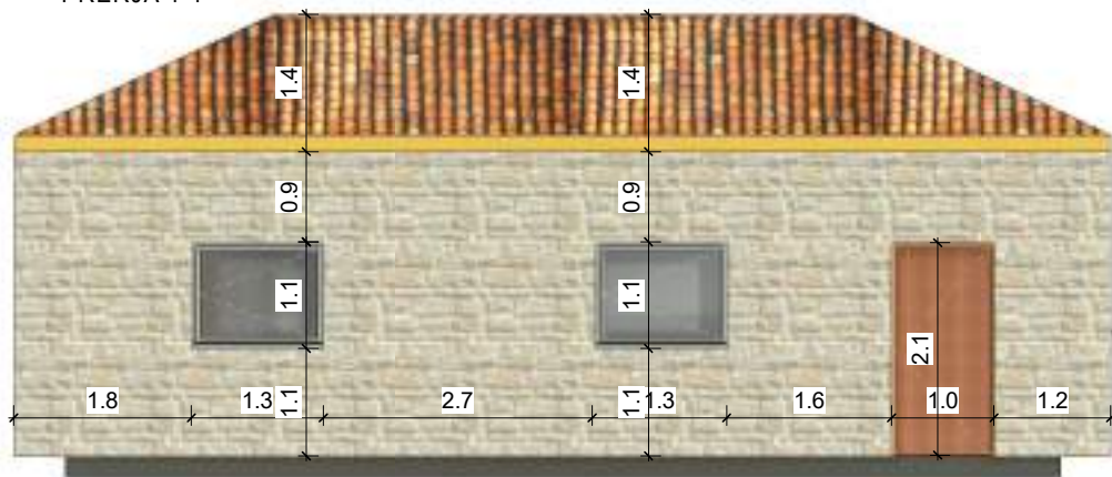
PRERJA 1-1
