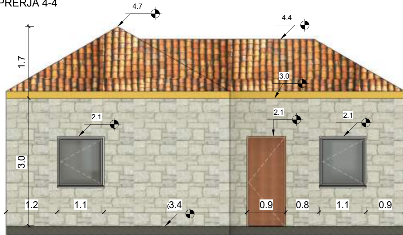
PRERJA 4-4
