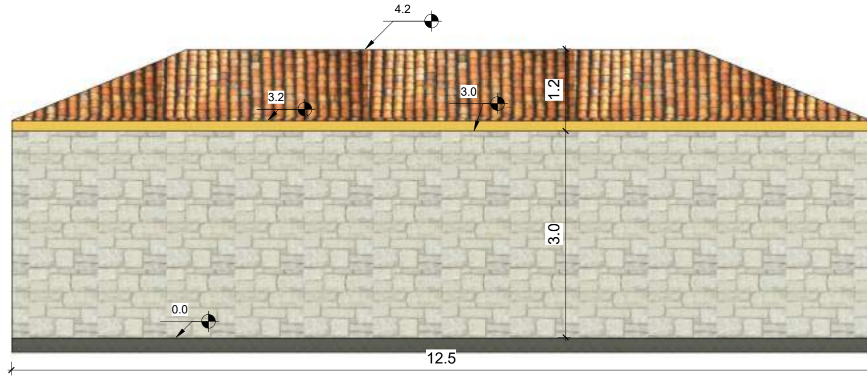
PRERJA 3-3
