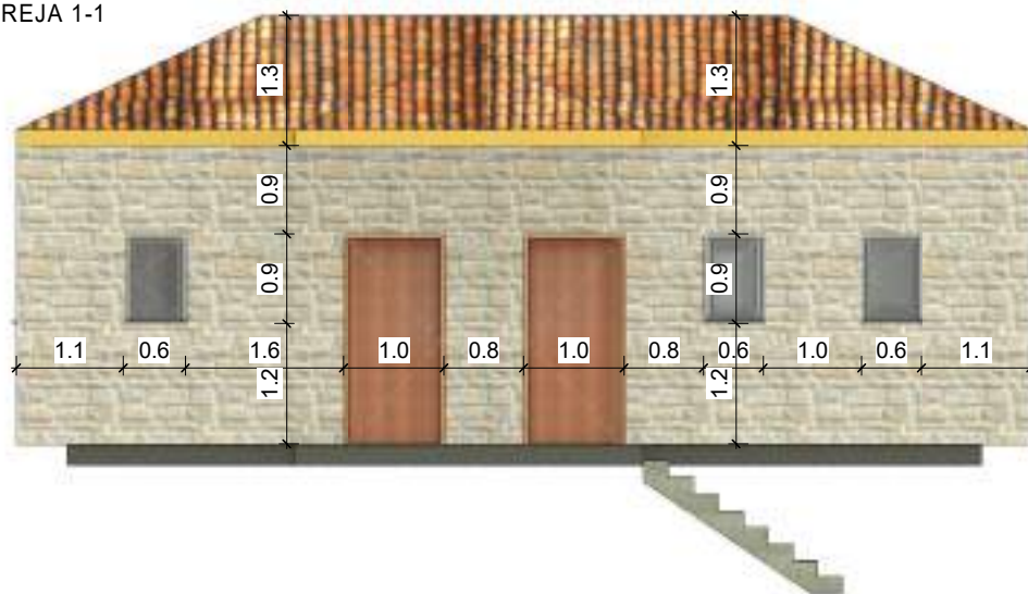
PREJA 1-1
