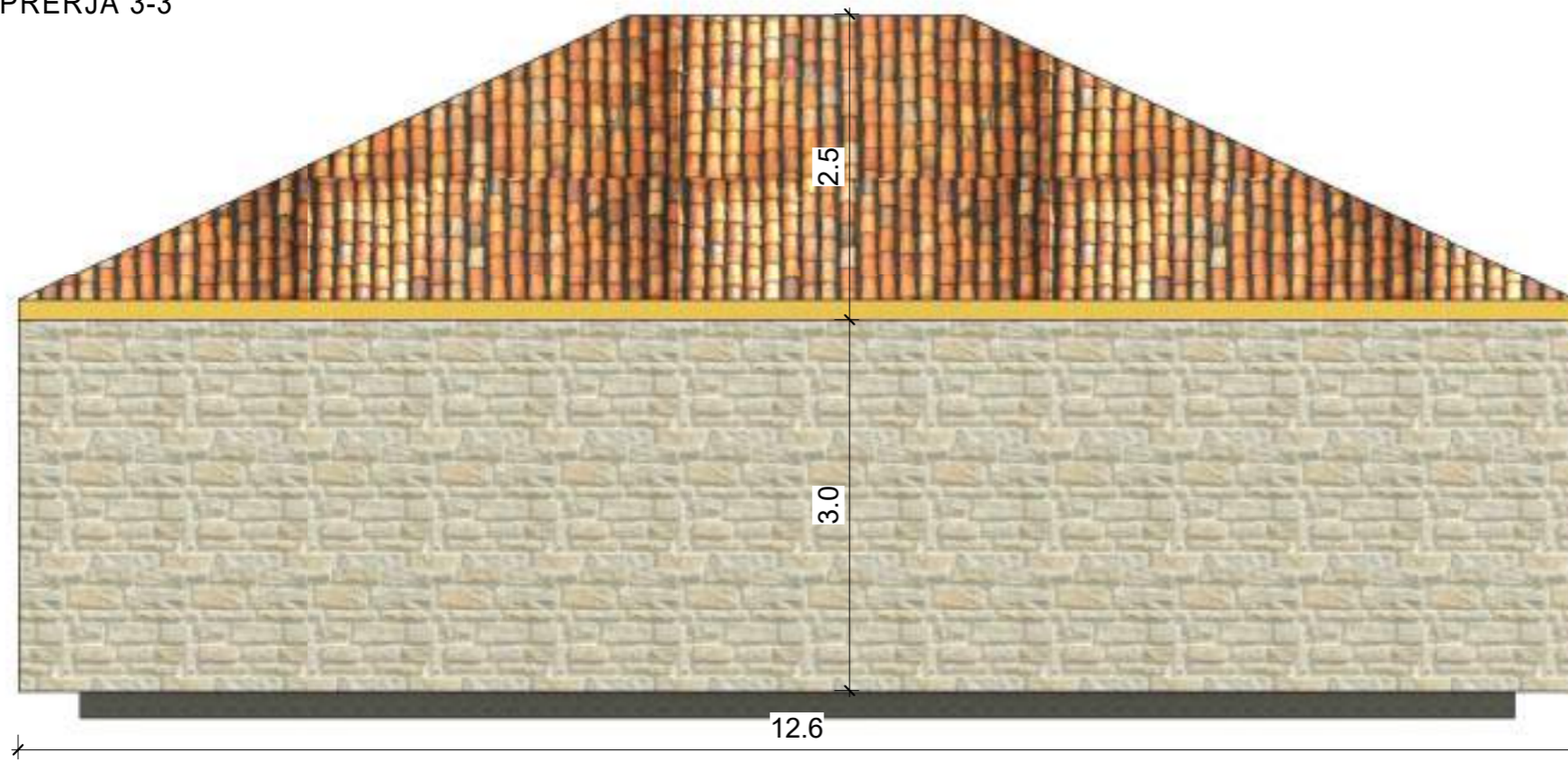
PRERJA 3-3
