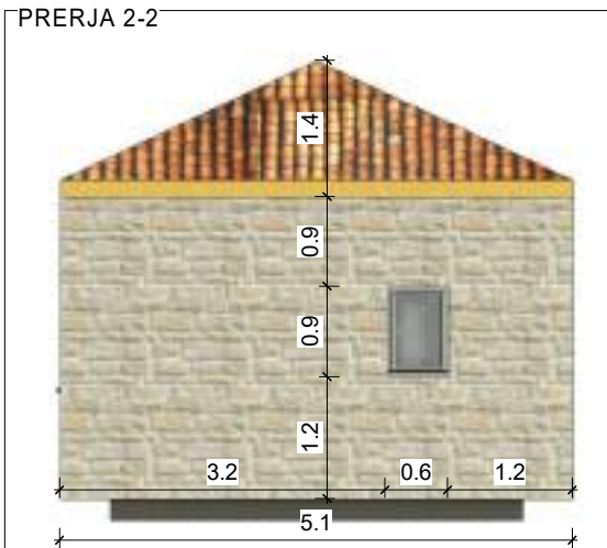
PRERJA 2-2
