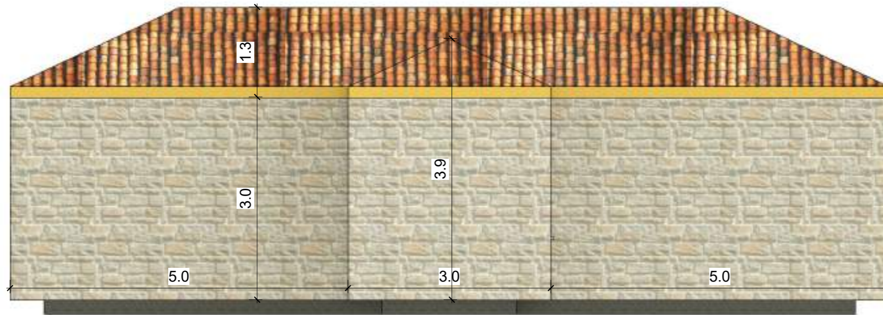
PRERJA 3-3
