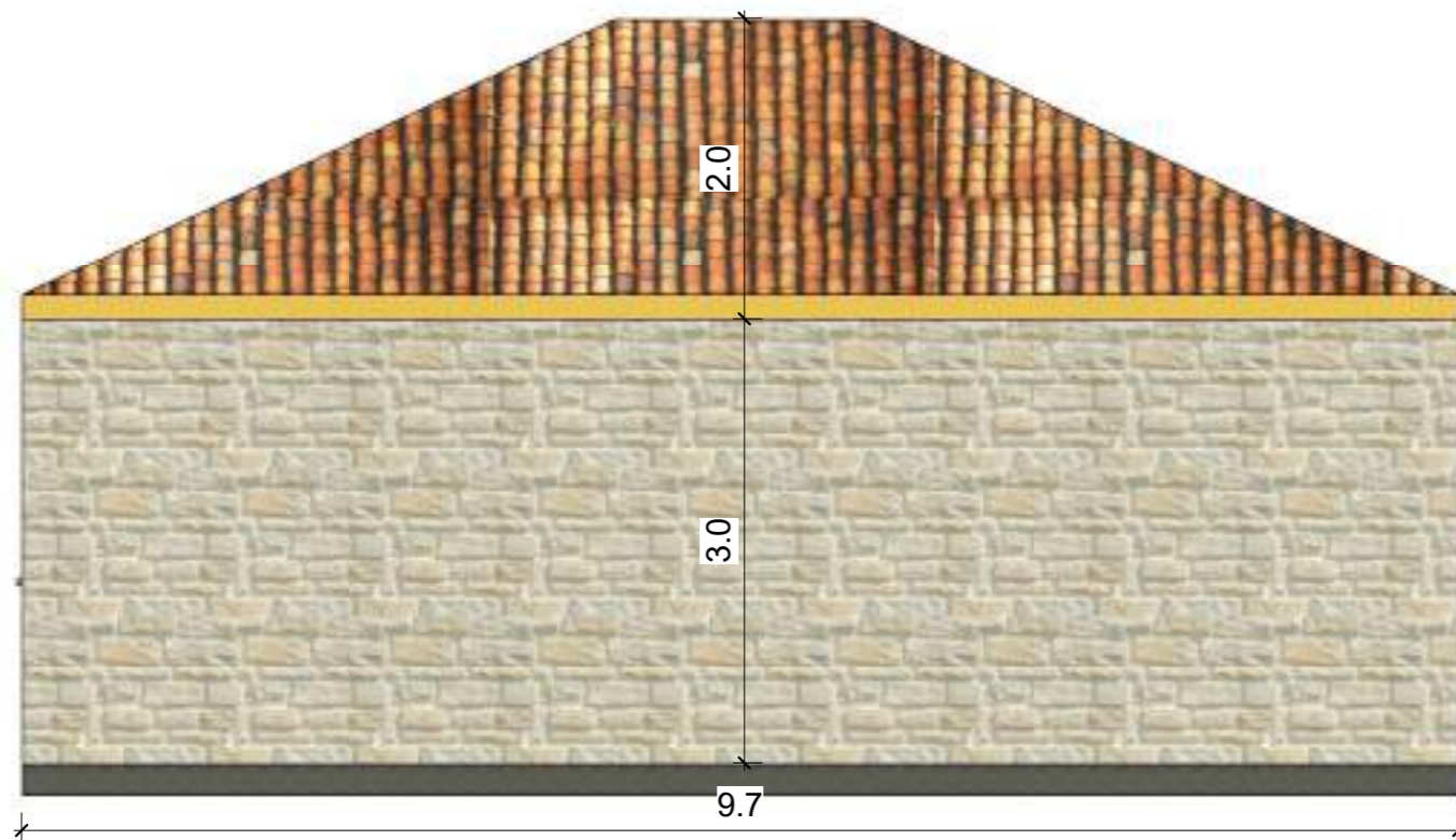
PRERJA 1-1
