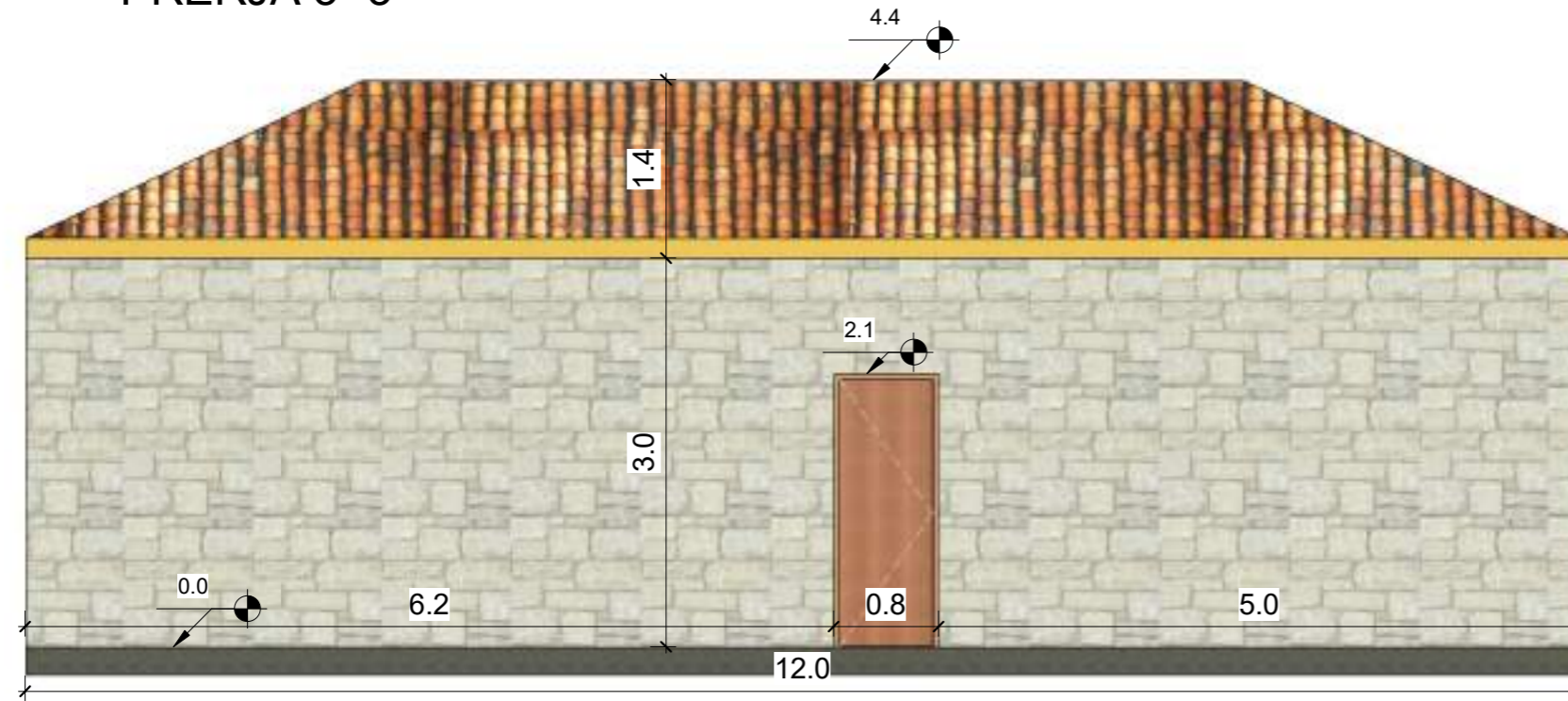
PRERJA 3 -3
