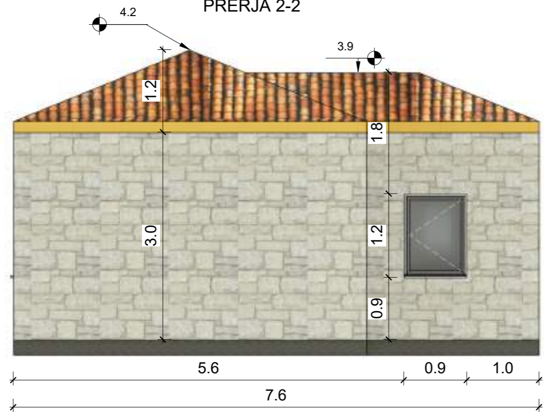
PRERJA 2-2
