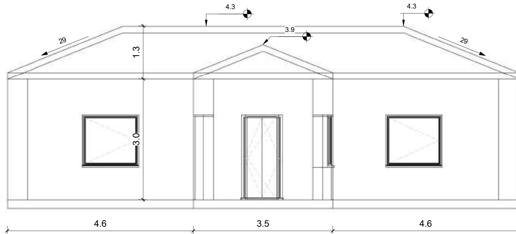
PRERJA 3-3
