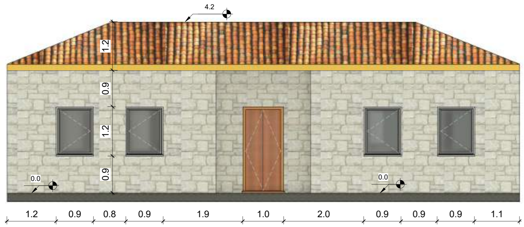
PRERJA 1-1
