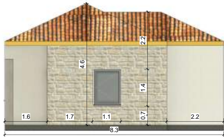
PRERJA 2-2
