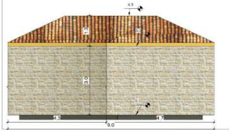
PRERJA 1-1
