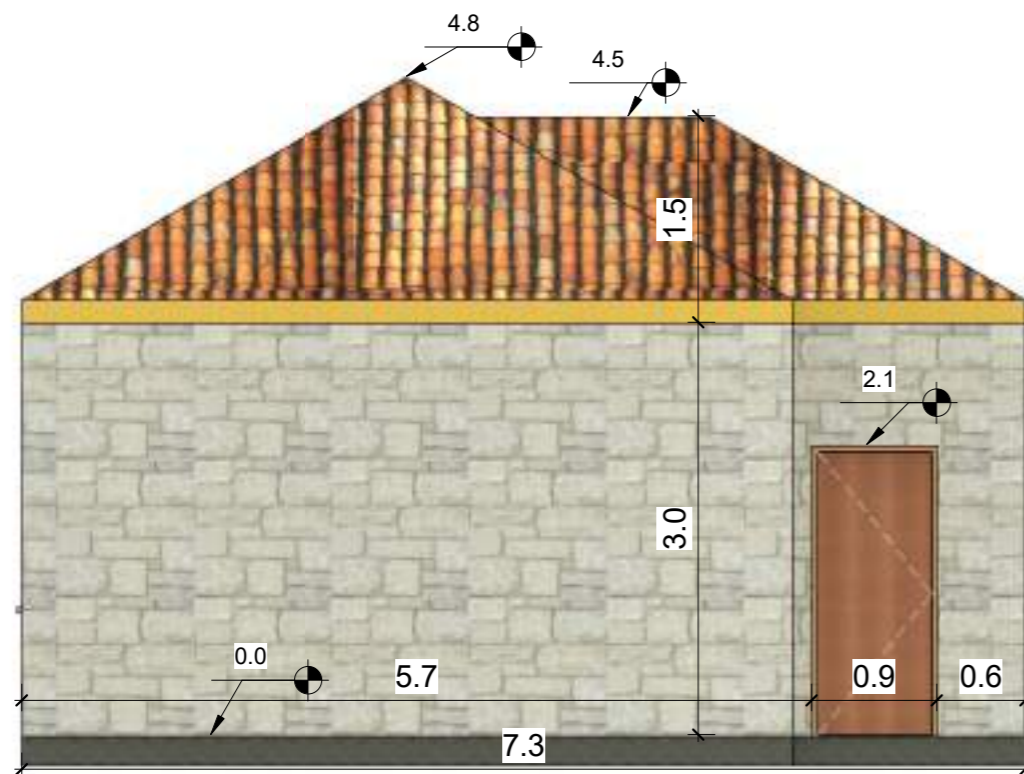
PRERJA 2-2
