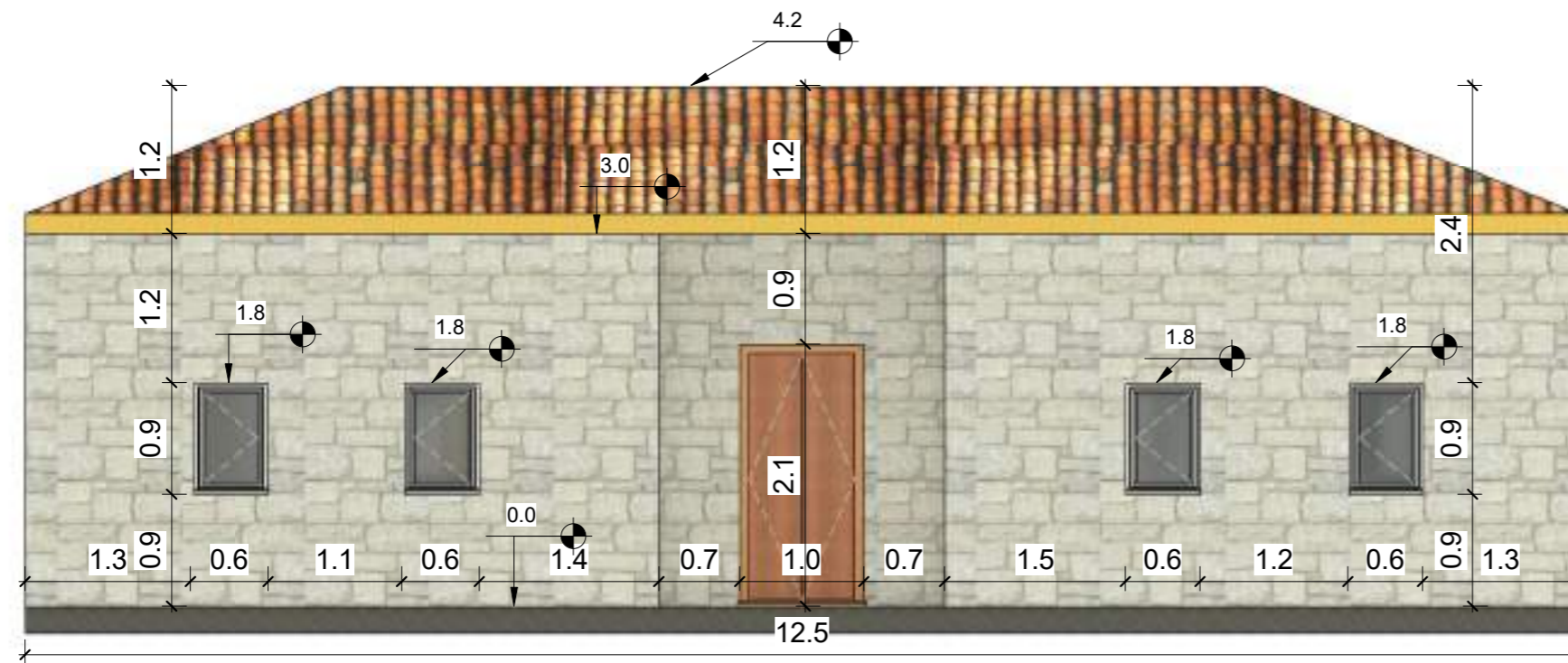
PRERJA 1-1
