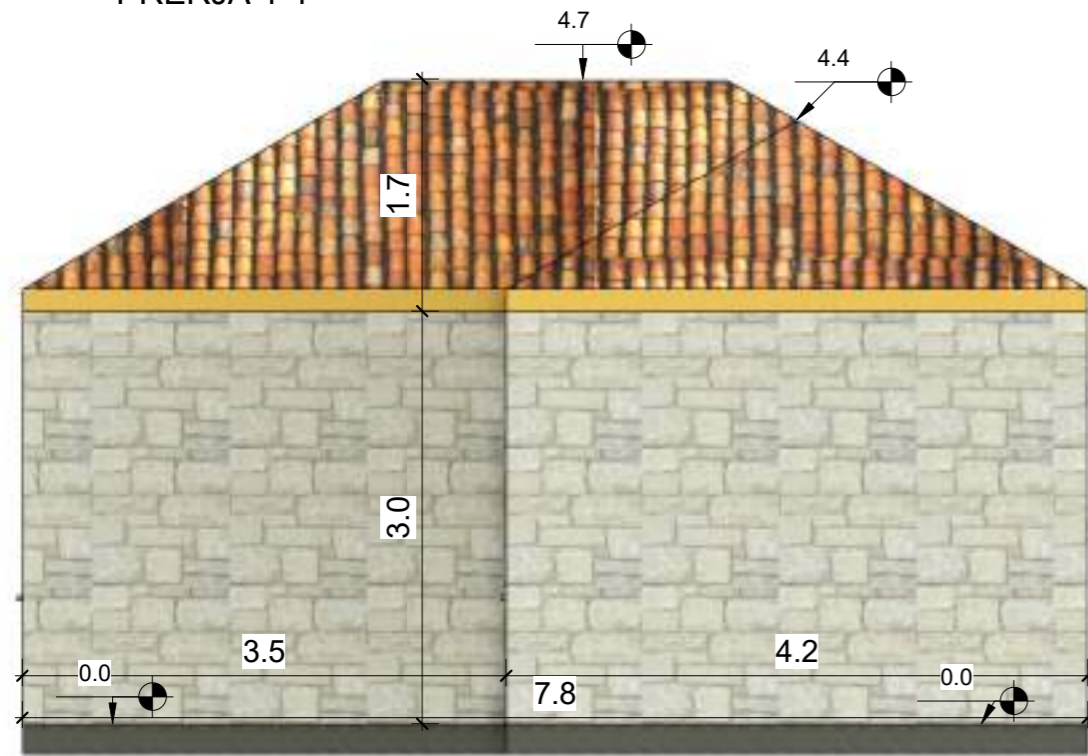
PRERJA 1-1
