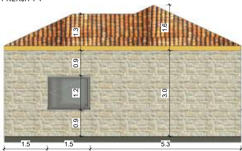
PRERJA 4-4
