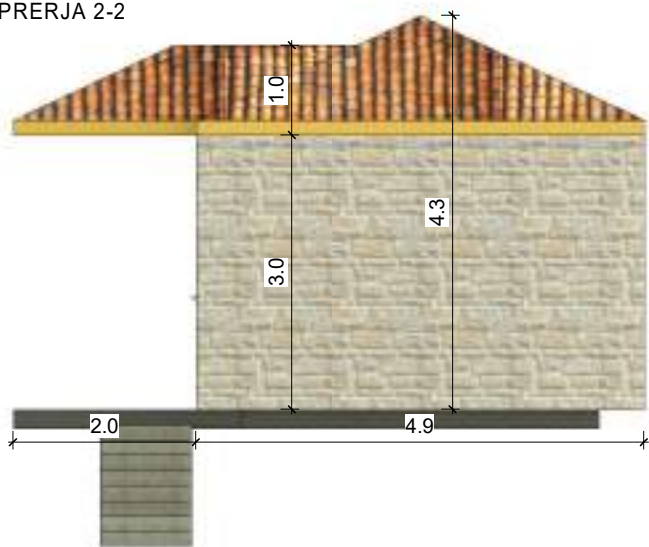
PRERJA 2-2
