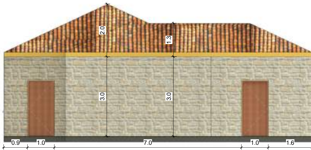
PRERJA 2-2
