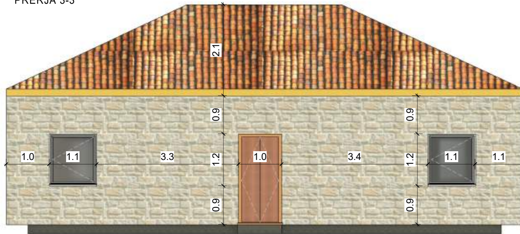
PRERJA 3-3
