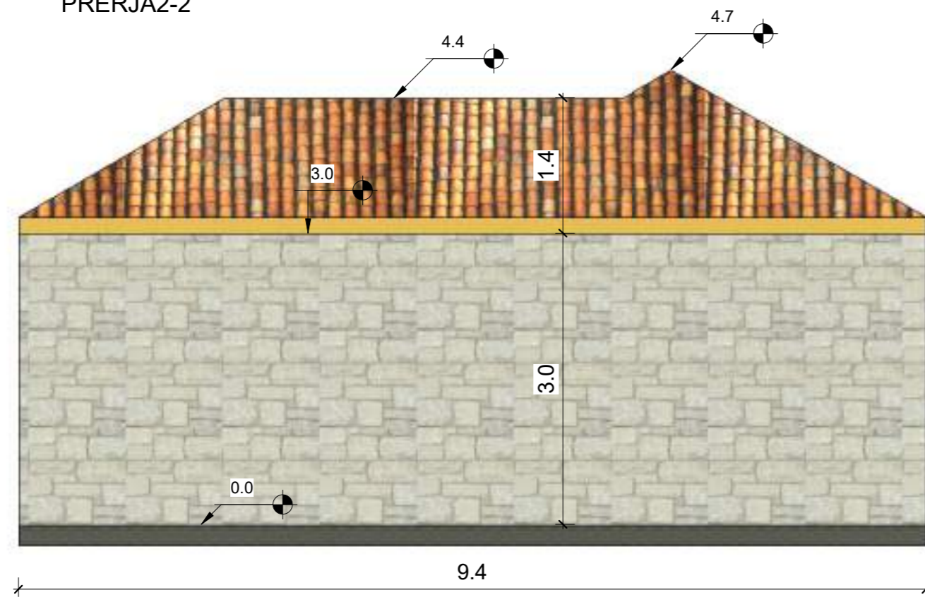
PRERJA2-2
