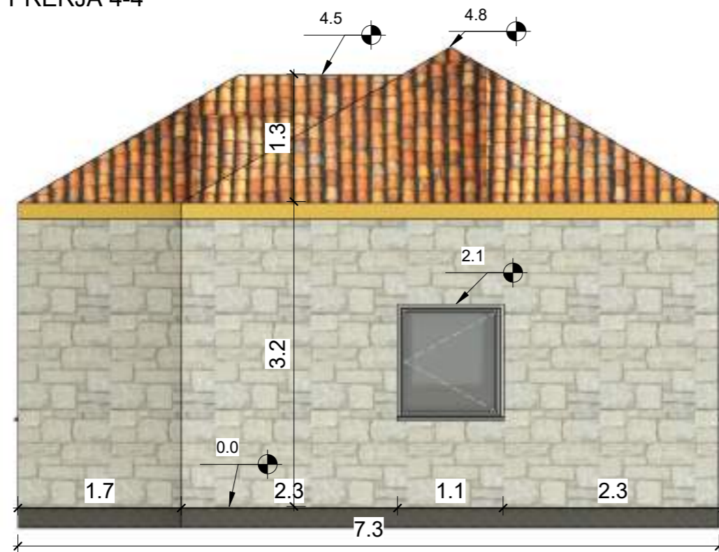
PRERJA 4-4
