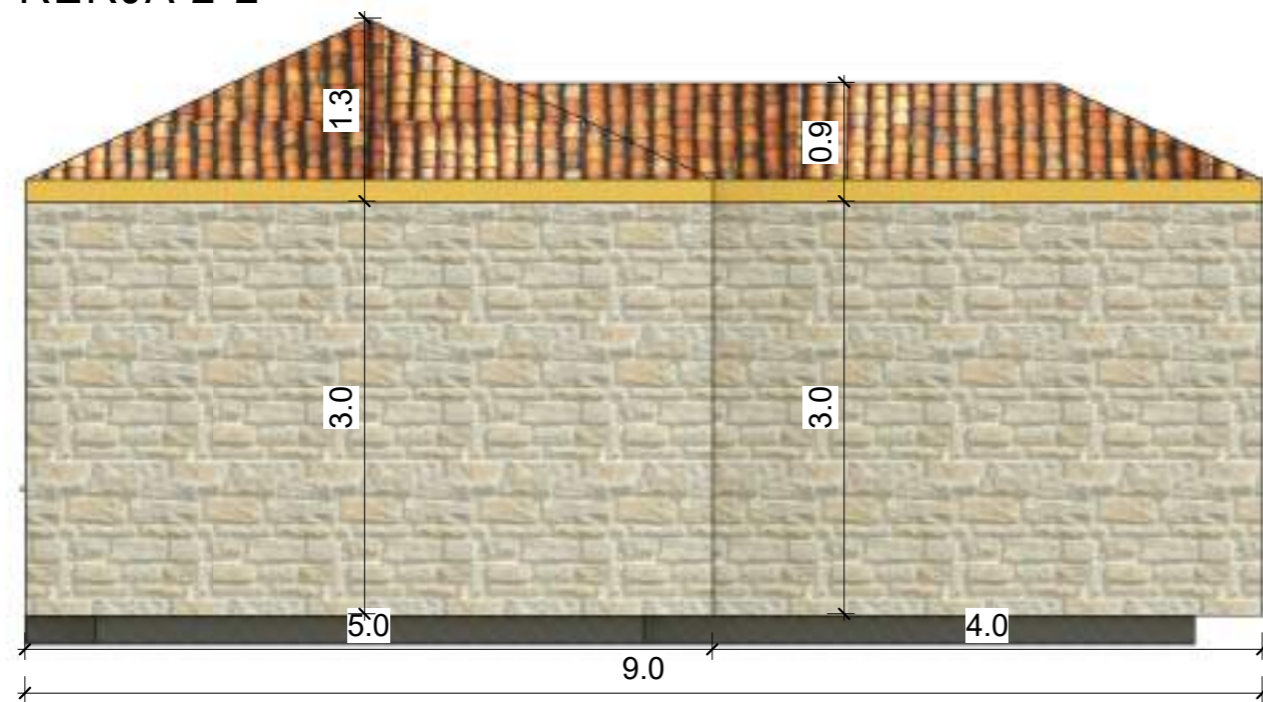
PRERJA 2-2
