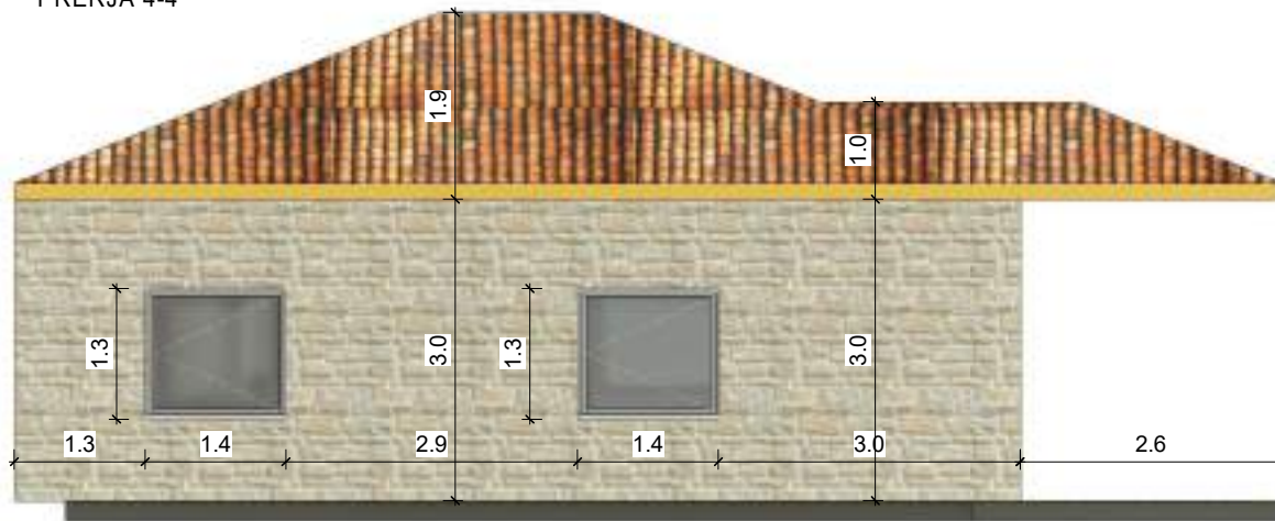
PRERJA 4-4
