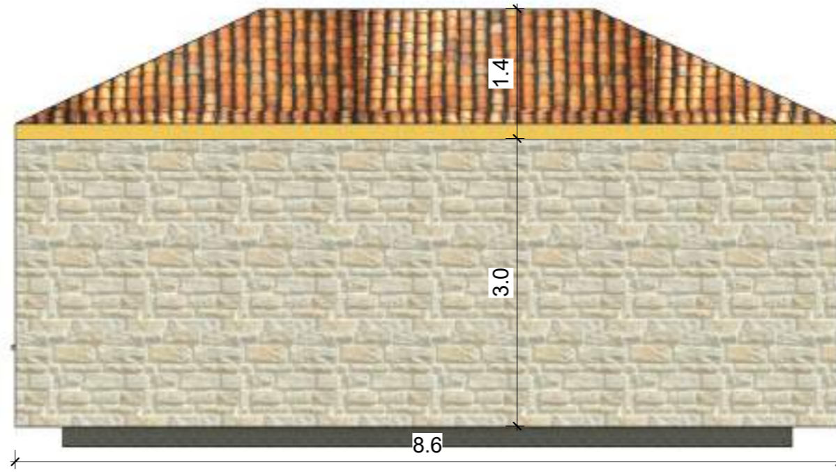
PRERJA 3-3
