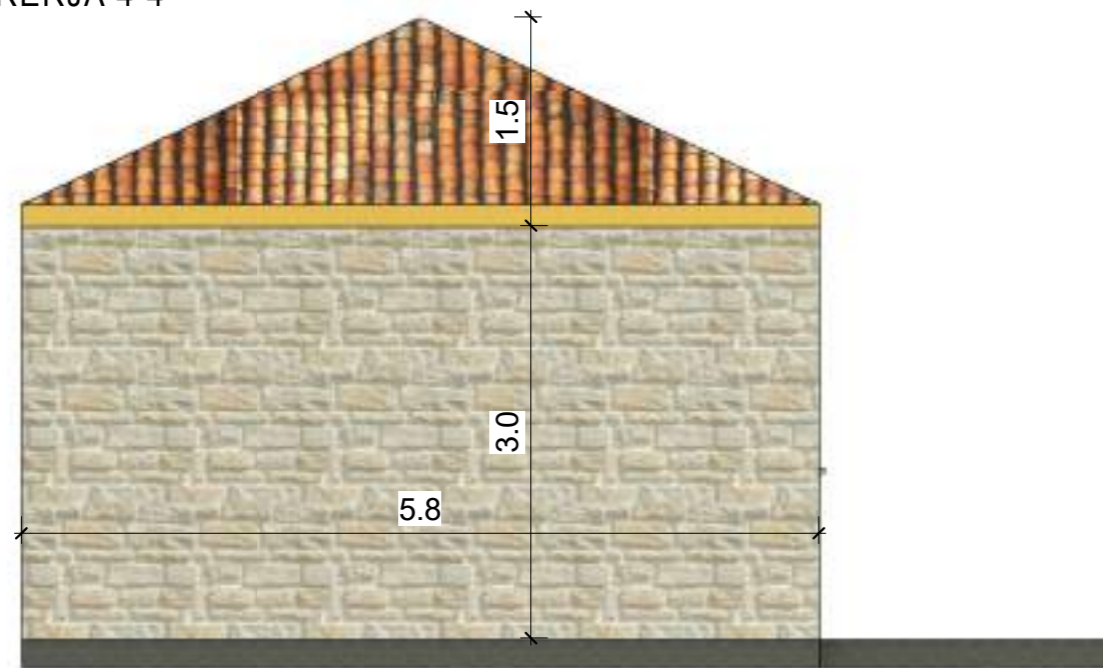
PRERJA 4-4
