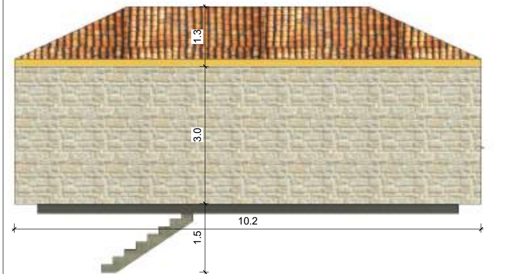
PRERJA 3-3
