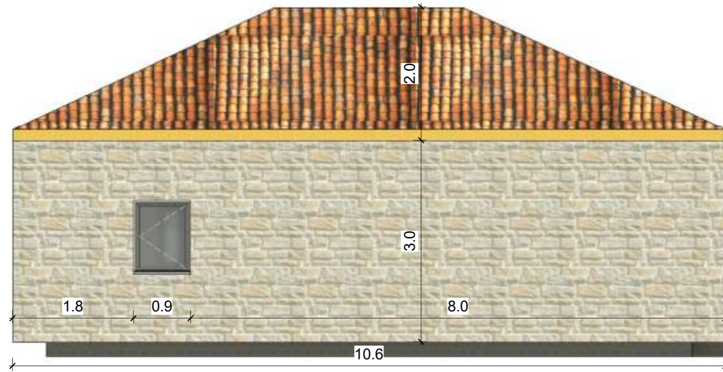
PRERJA 3-3
