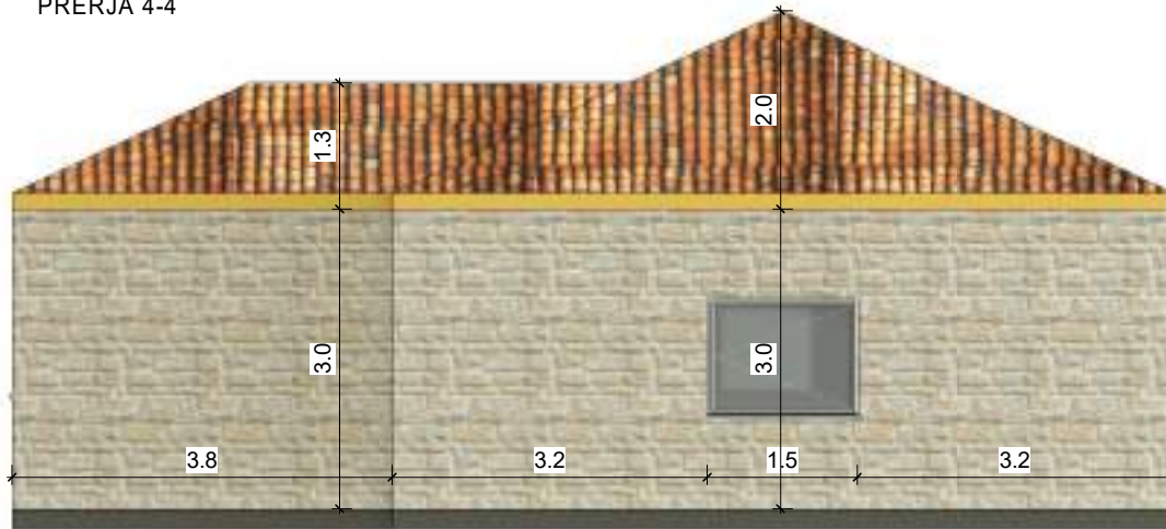
PRERJA 4-4
