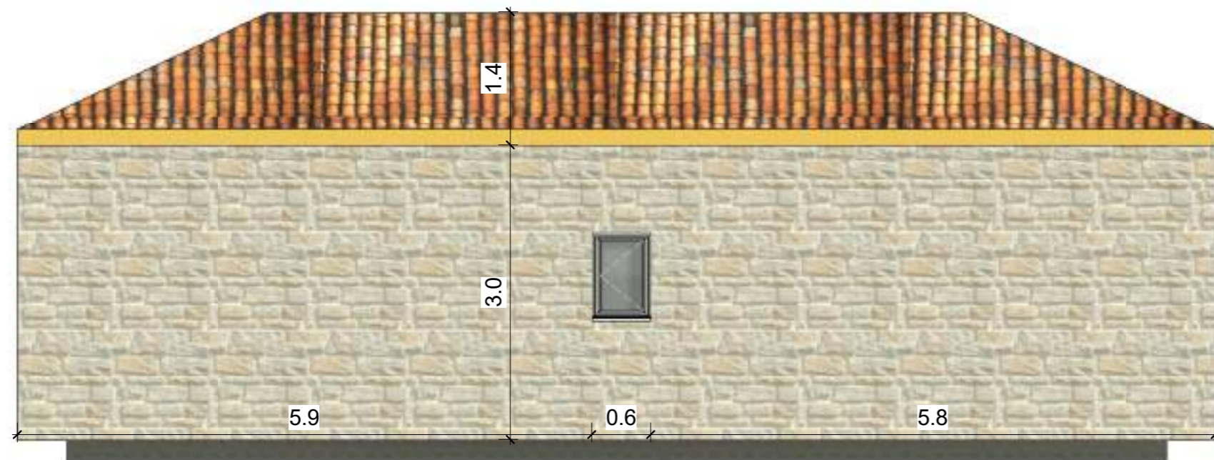
PRERJA 3-3
