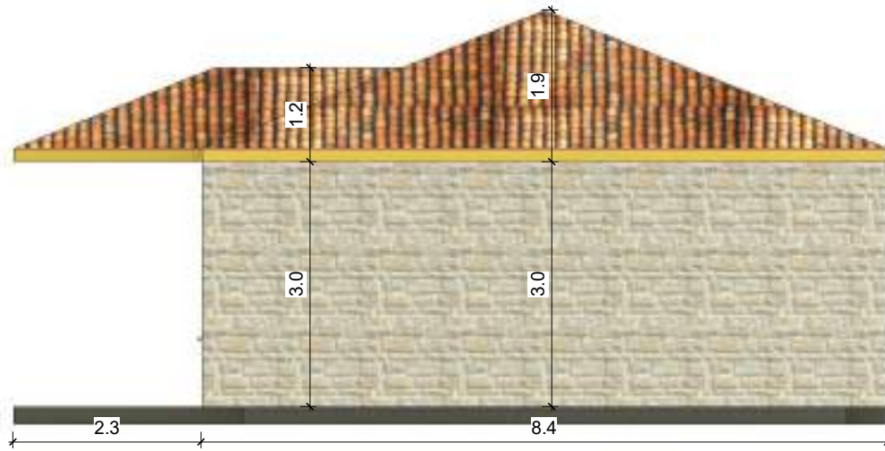
PRERJA 4-4
