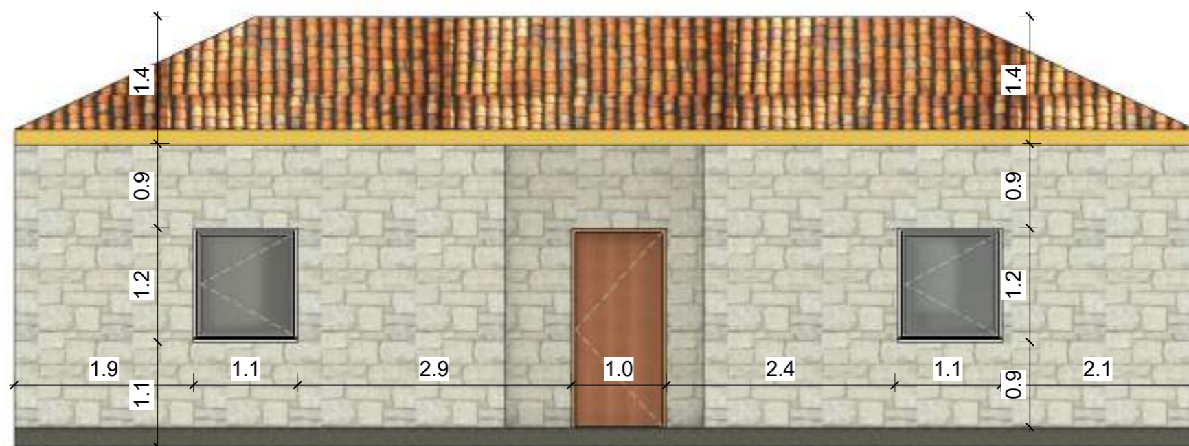
PRERJA 1-1
