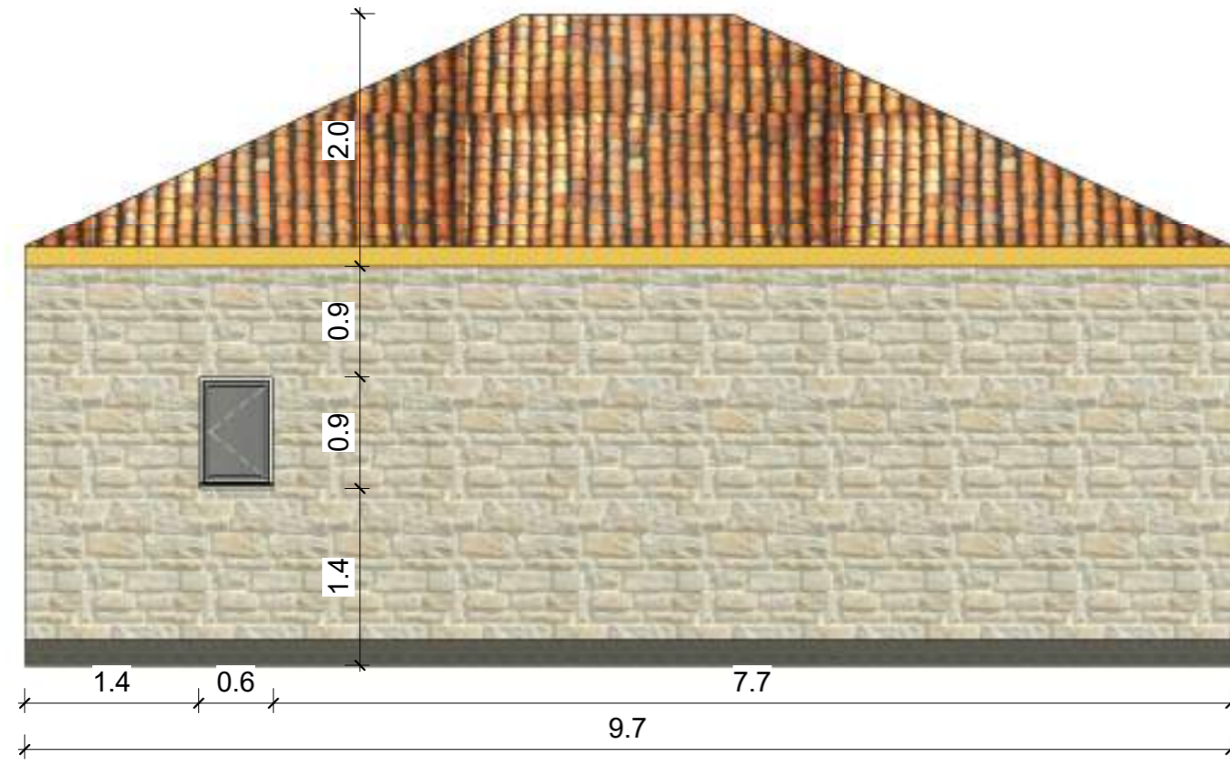
PRERJA 3-3
