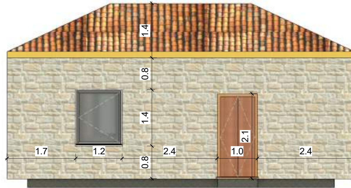
PRERJA 1-1
