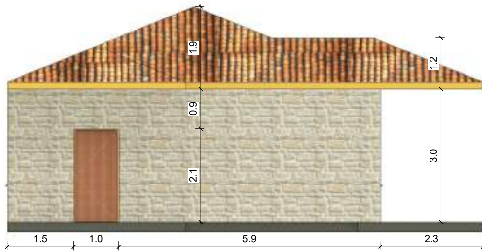
PRERJA 1-1
