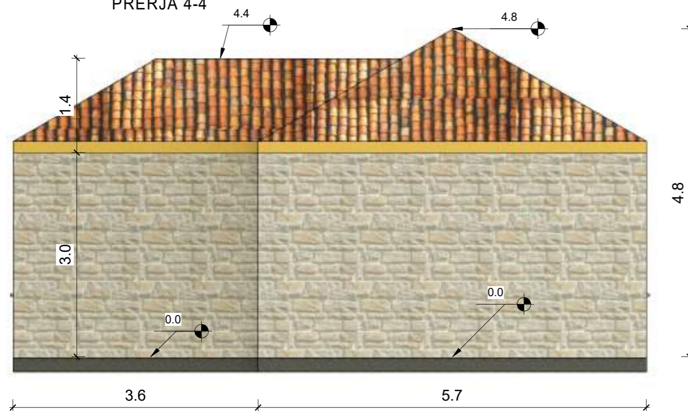
PRERJA 4-4
