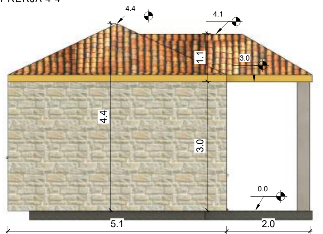
PRERJA 4-4
