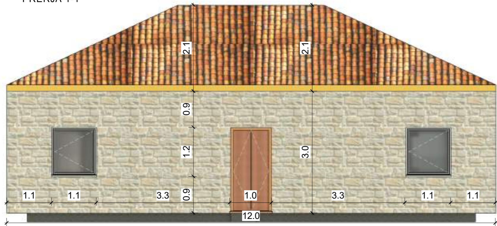
PRERJA 1-1
