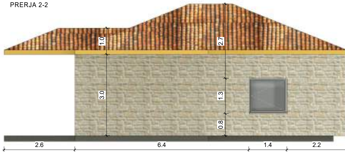
PRERJA 2-2
