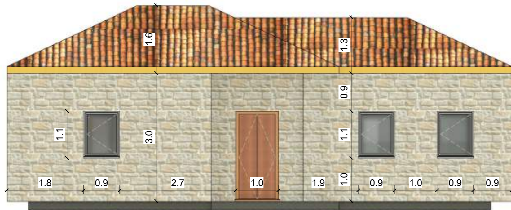
PRERJA 3-3
