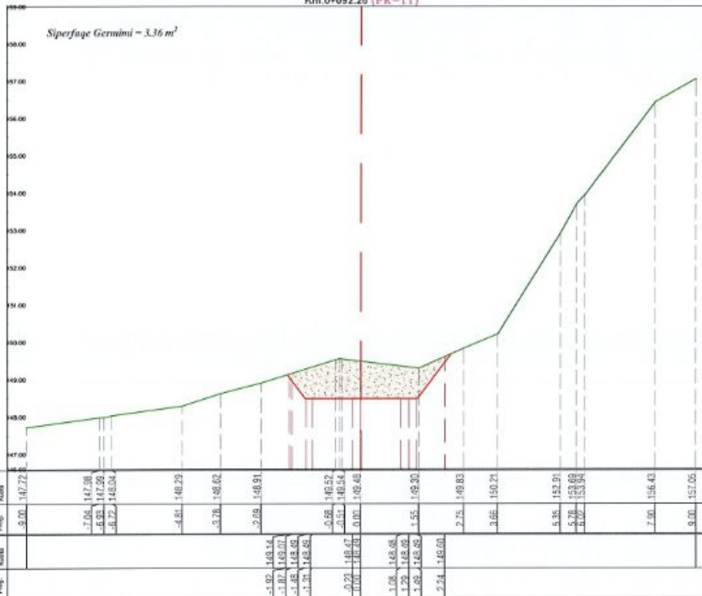
Km 0+092.26 (PK-11)
