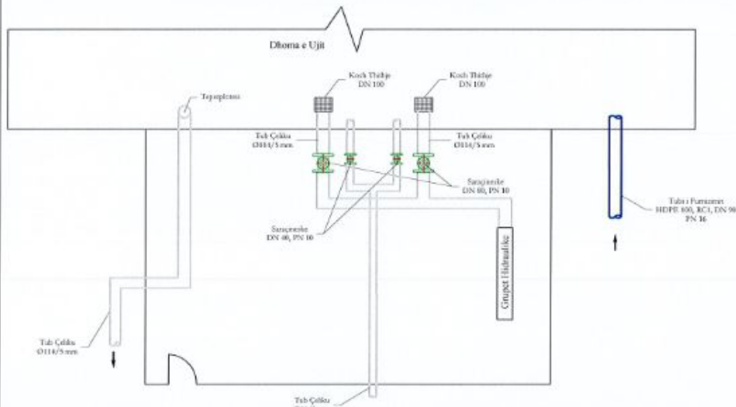
SKEMA HIDRAULIKE E DEPOS
