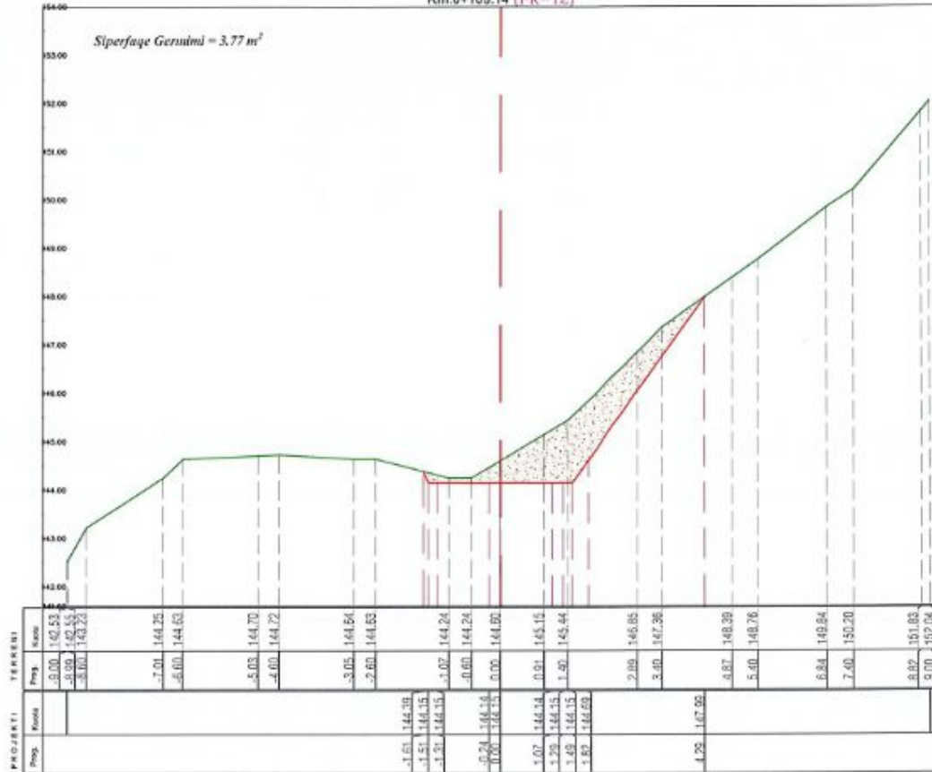
Km 0+105.14 (PK-12)
