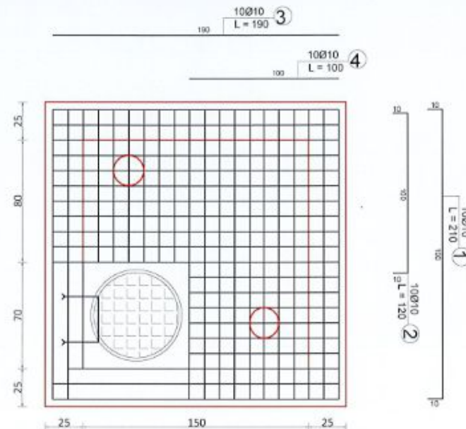
T-1 SH 1:25
