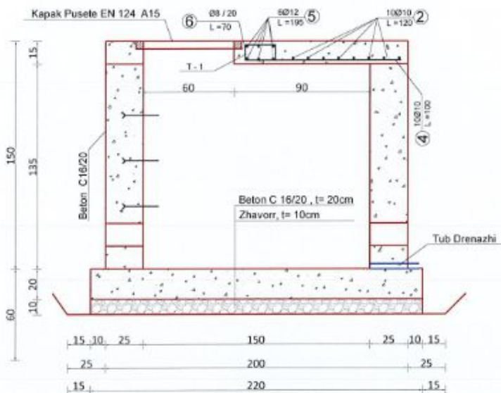
PRERJA A-A SH 1:25
