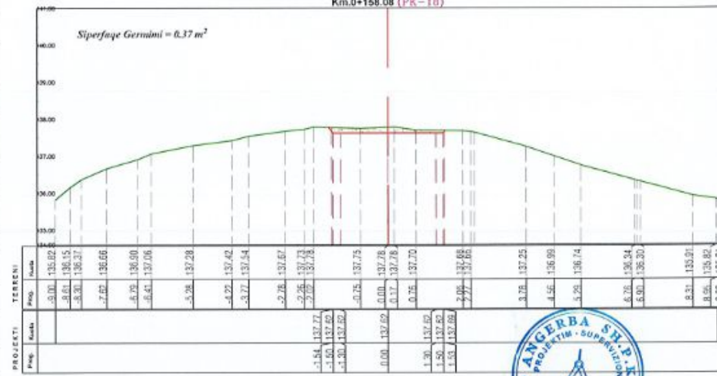
Km.0+158.08 (PK-18)
