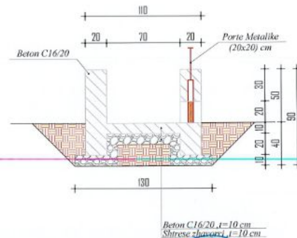
PRERJA A-A SH. 1:25
