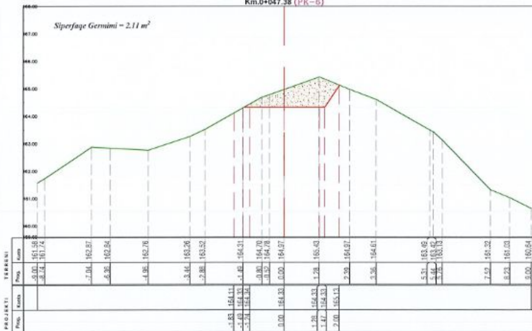
Km.0+047.38 (PK-6)
