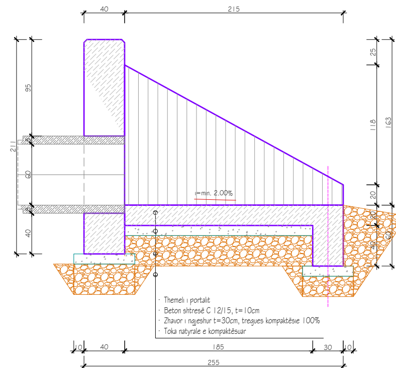
Prenja 1-1 e Munt b/a të portalit të pjerrët të tombinos Ø600mm, Sh. 1:25
