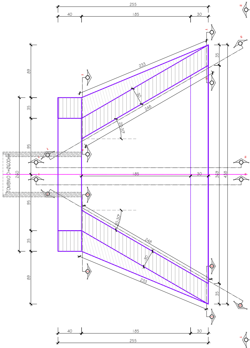
Plani i Munt b/a të portalit të pjerrët të tombinos Ø600mm, Sh. 1:25
