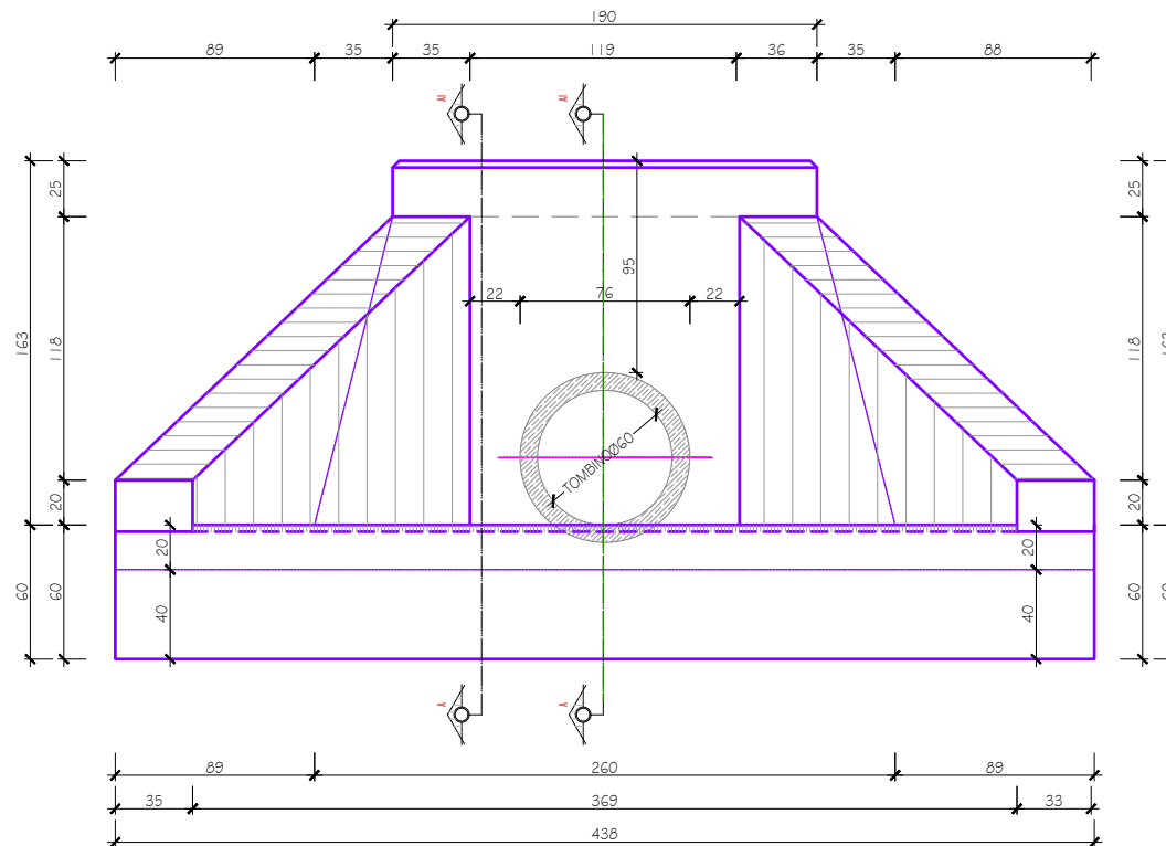
Prenja 2-2 e Munt b/a të portalit të pjerrët të tombinos Ø600mm, Sh. 1:25
