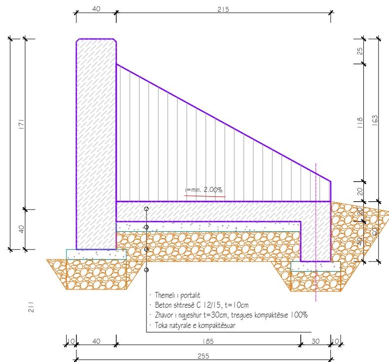
Prenja 2-2 e Munt b/a të portalit të pjerrët të tombinos Ø600mm, Sh. 1:25
