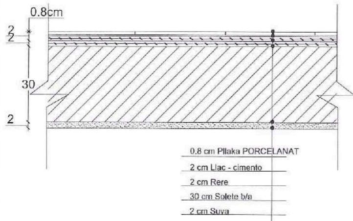
DETAJ I SOLETES NDERKAT
