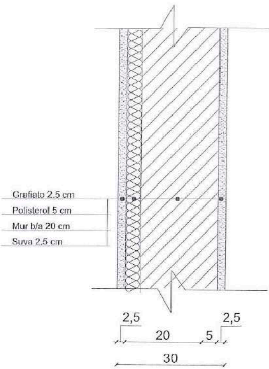
DETAJ I MURATURES SH - 1:12
