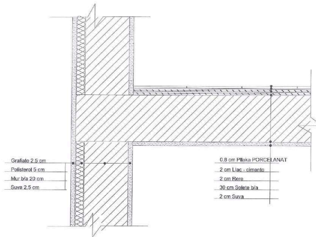
DETAJ I MURATURES + SOLETE - 1:12
