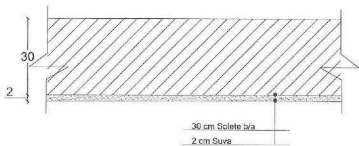
DETAJ I TAVANIT SH - 1:10
