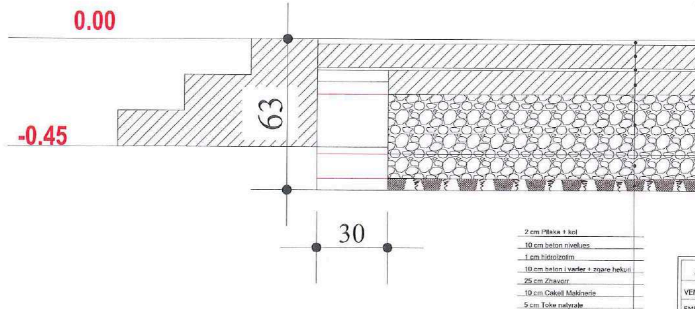
DETAJ I SOLETES KUOTA 0.00
