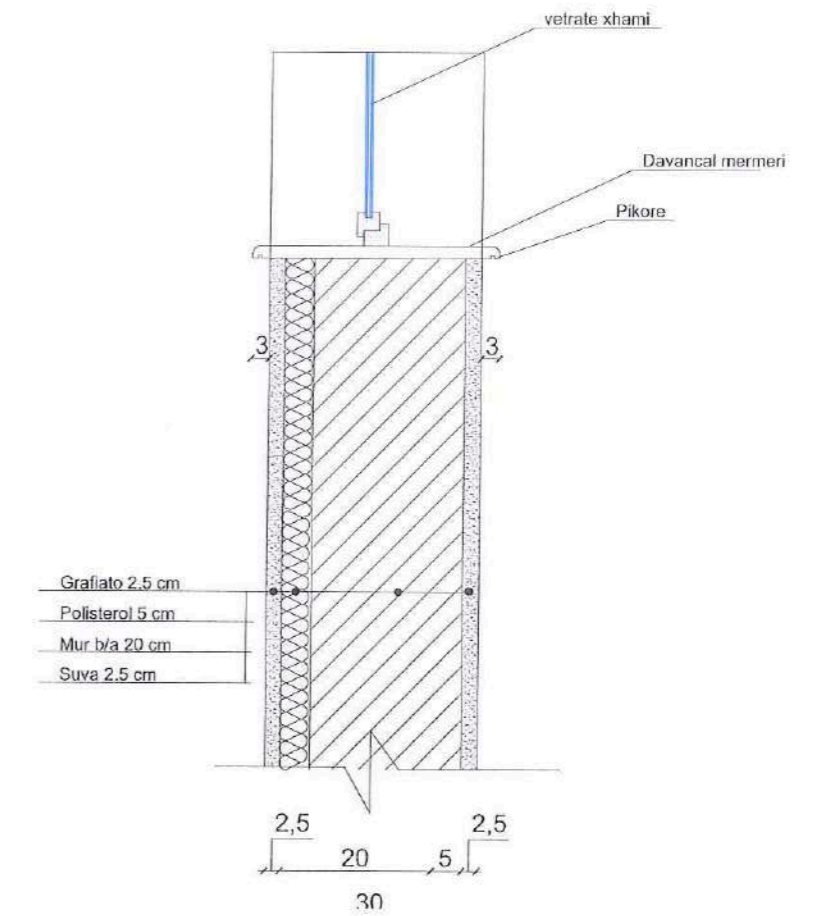
DETAJ I MURATURES + DRITARE - 1:12
