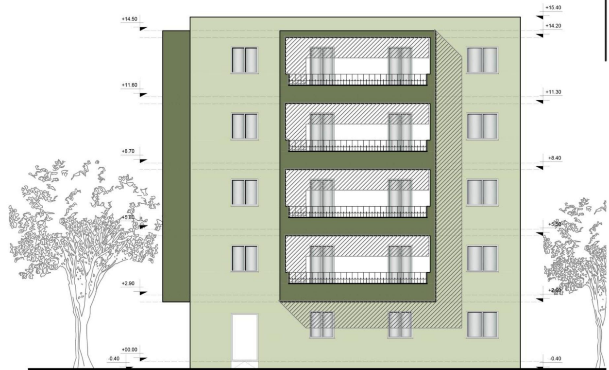
Fasada nga Lindja Shk. 1:100
