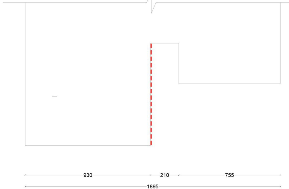
Planimetria
