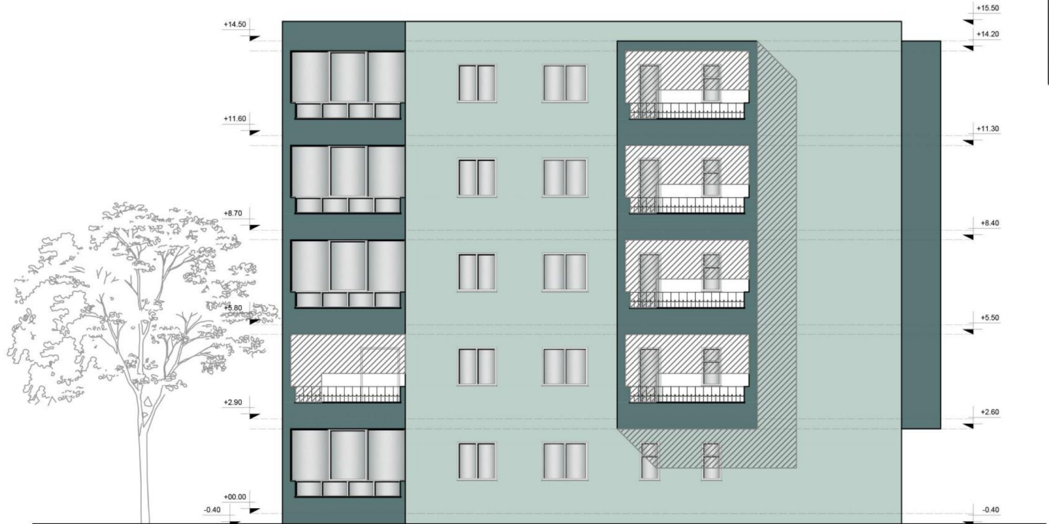
Fasada nga Jugu
