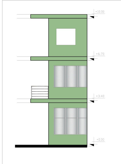
FASADA NGA LINDJA SHKALLE 1:100
