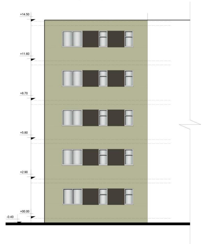
Shk. 1:100
