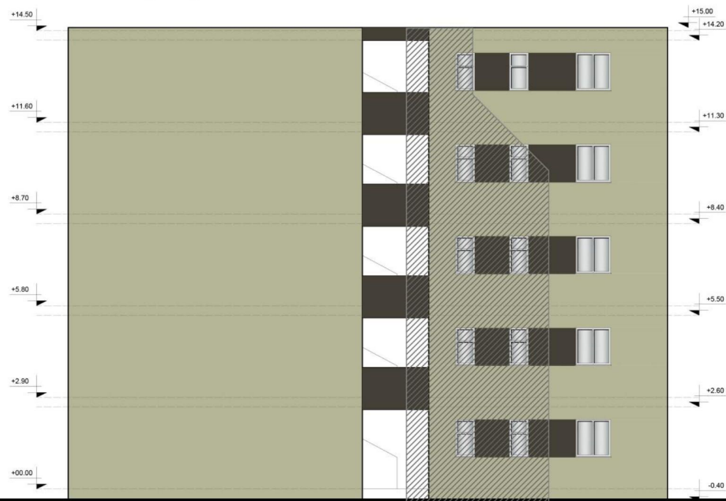
Fasada nga Jugu
