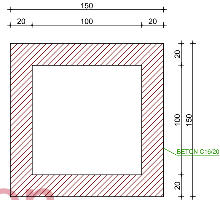
PLANIMETRI SH 1:20
