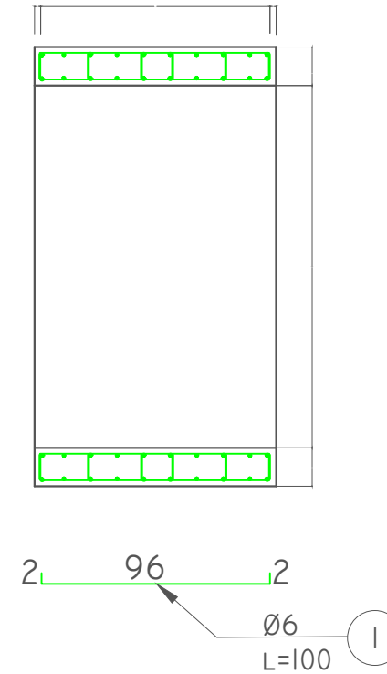
SASIA E HEKURIT PER NJE TUB
