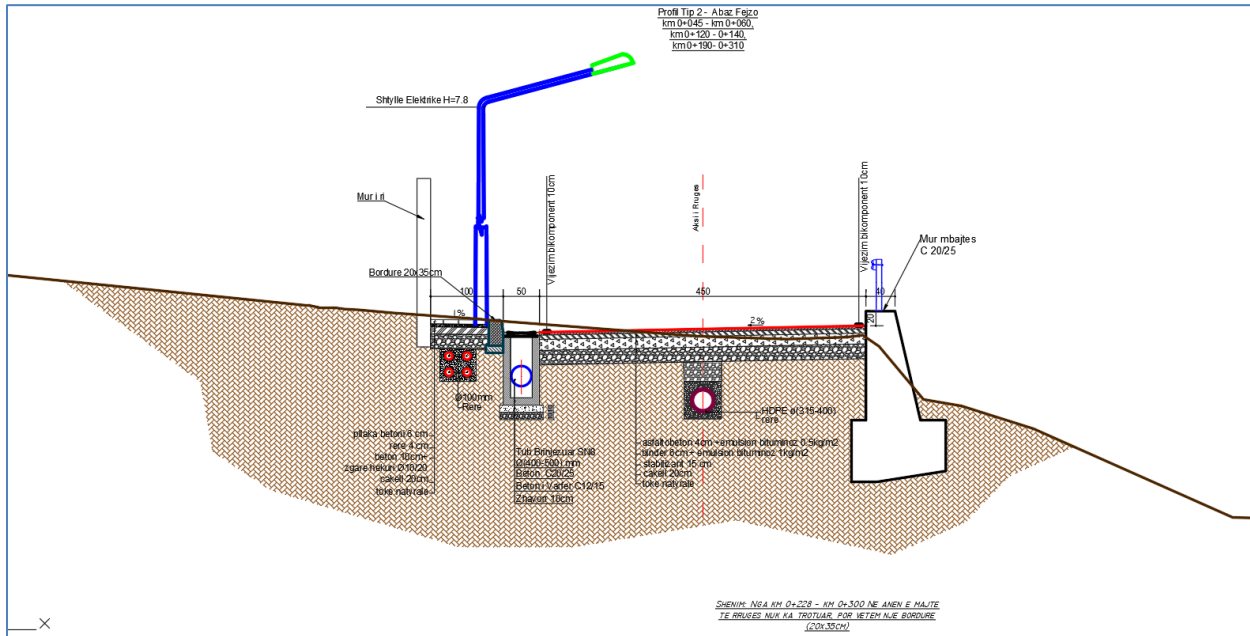
Profili Terthor Tip
