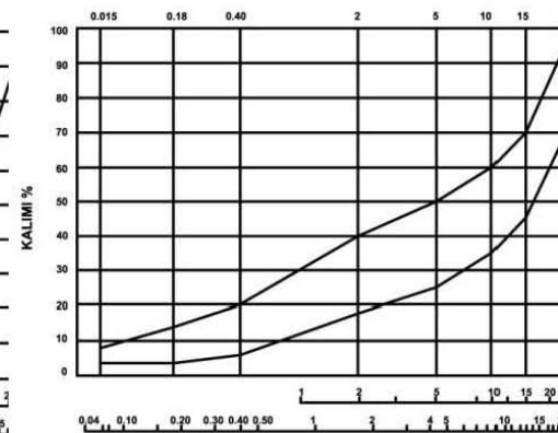
Figura 3: Perzierje granulometrike per shtresen bazë
