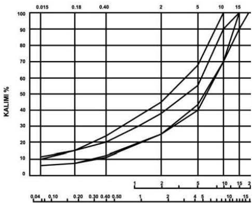
Figura 1: Perzierje granulometrike per shtresen e pendorimit D_{max}=20 D_{max}=15
