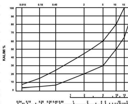
Figura 2: Perzierje granulometrike per shtresen e lidhjes
