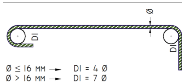
Fig. 1 – Zgjedhja e diametrit të mandrinës për kthimin e shufrave në varësi të diametrit të shufrave
