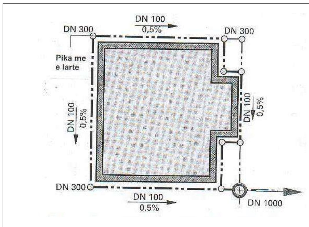
Figura Nr. 2 - Mënyra e vendosjes se tubave të drenazhimit
