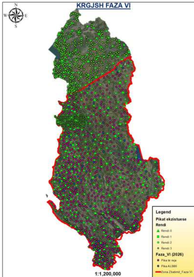
Fig. 4.1. Pozicionimi i dendësimit të mëtejshëm të pikave të Rrjetit Gravimetrik të Rendit III, në pjesën qendrore dhe jugore të Shqipërisë (pikat me ngjyrë rozë dhe blu).
