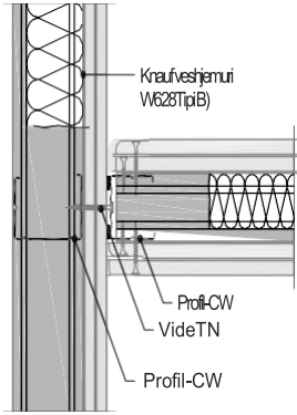
W112-A7 Bashkimi meveshjenemuit
