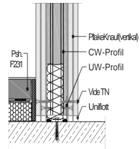
W112-VU1 Bashkimi ne dymsheme
