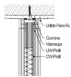
W112-VO1 Bashkimi i murit mesletenelavan
