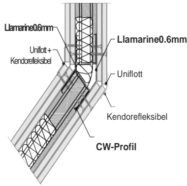
W112-D2 Kendi i gjere CW+kendorefleksibel
