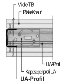
W112-VU1 Bashkimi ne dymsheme
