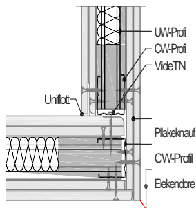
W112-D1 Detaj i kendit drejte
