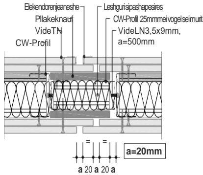
W112-BFU1 Fugedilataoni nerastet kur muri eshte me i gjatese 15m
