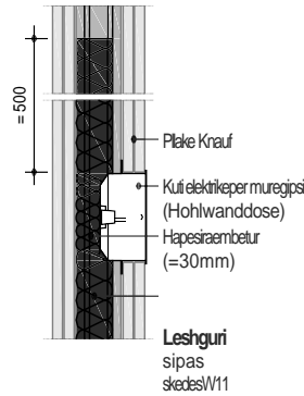
W112BS-ELT5 Kufi elektrike
