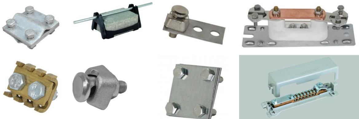
Figura 10-5: Morseta, shkëputës tokëzimi, suport dhe zbarë ekuipotenciale
