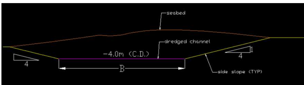
Fig. 4. Profili tërthor tip i thellimit të tabanit të basenit (e propozuar)
