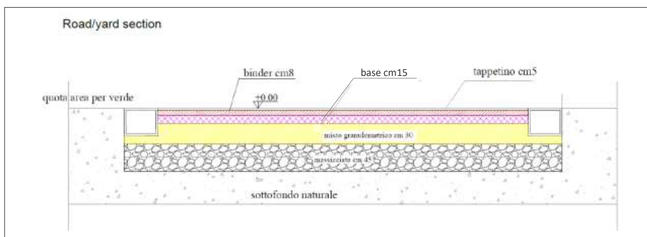
Fig. 5. Profili tërthor tip i rrugës auto (e propozuar)
