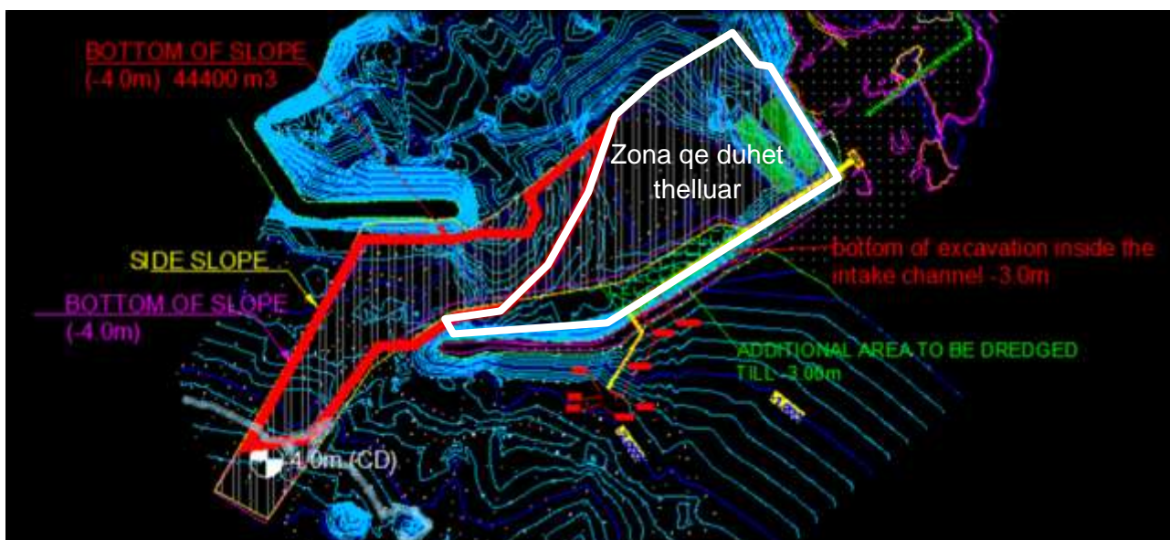
Fig.3. Planimetria e zonës që duhet thelluar e konturuar me ngjyrë të bardhë (e propozuar).
