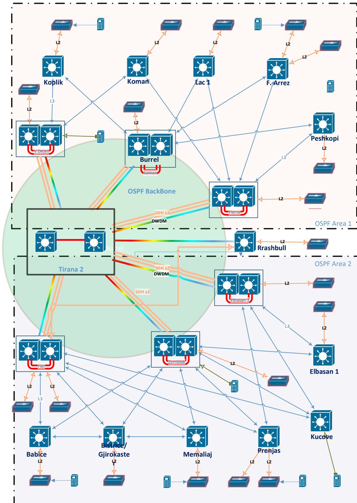
Figura 2 Topologjia e rrjetit Star - partial mesh
