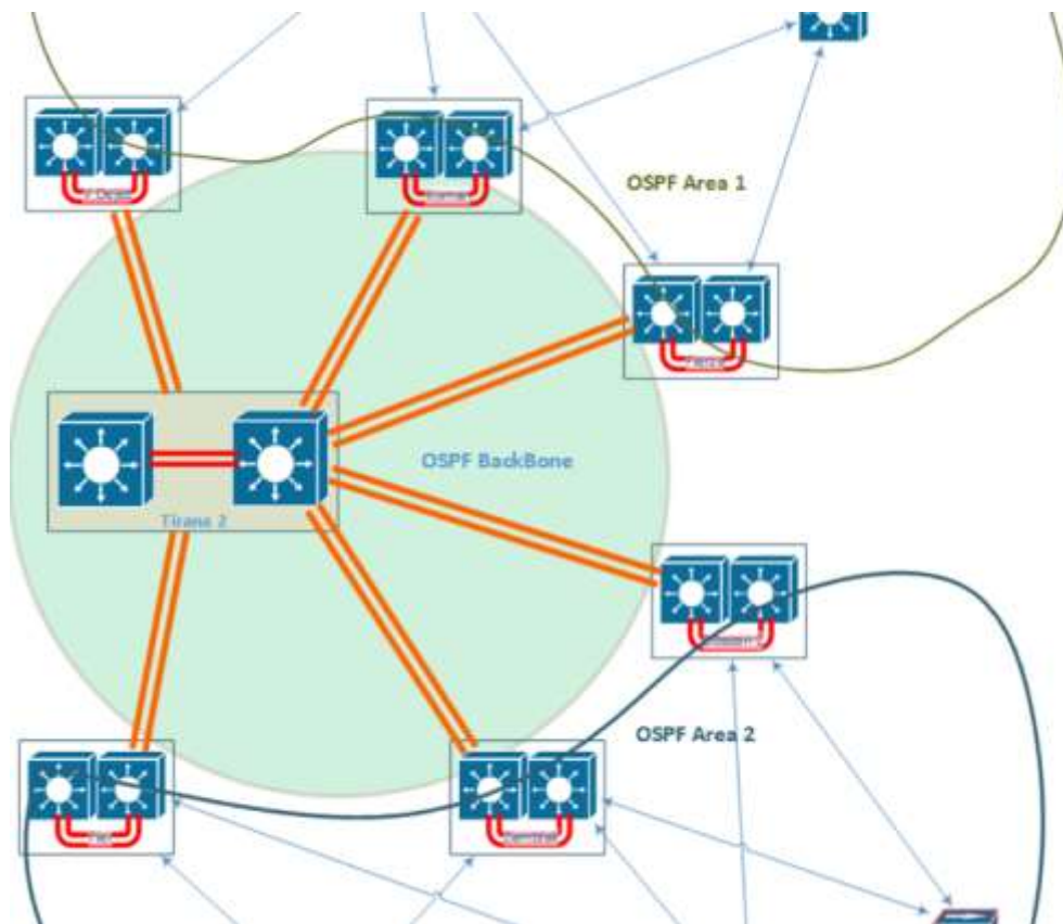
Figura 4 OSPF BackBone dhe kufiri me Area 1 dhe Area 2
