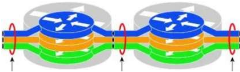
Figura 3 Paraqitja skematike e një switchi për instanca të ndryshme rutimi
