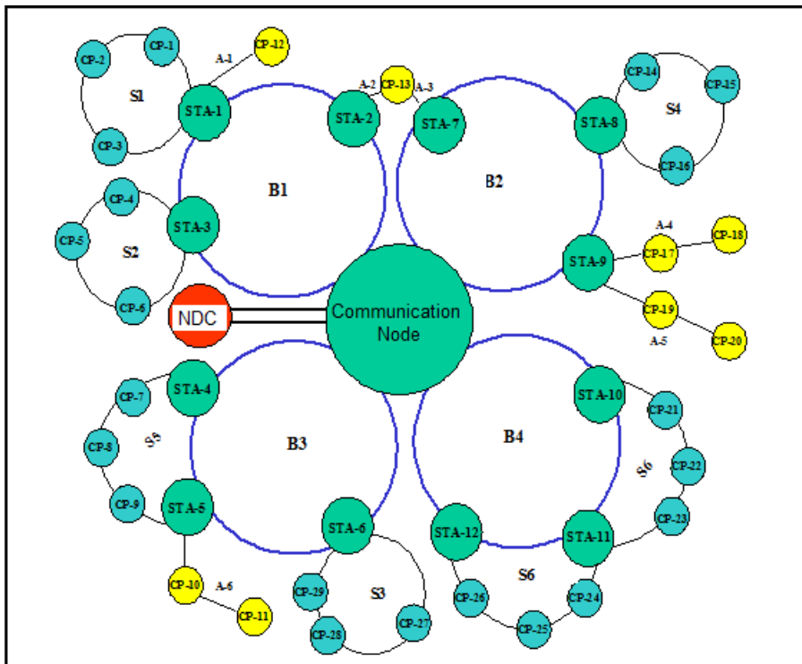
Figura 1 Arkitektura e Rrjetit të Komunikimit
