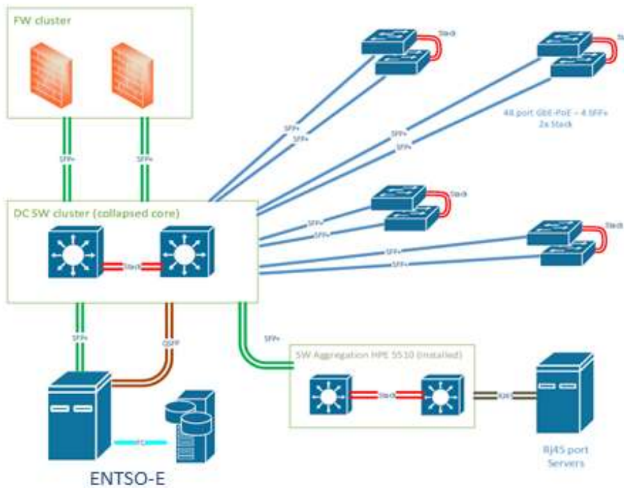
Figura 1 Topologjia e rrjetit Star - partial mesh
