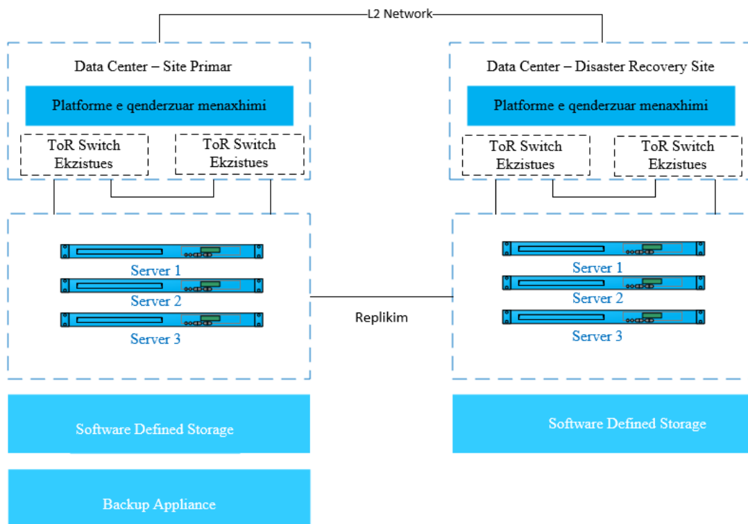
Fig. 1 – Paraqitje skematike e ambientit primar dhe sekondar te infrastruktures hostuese
