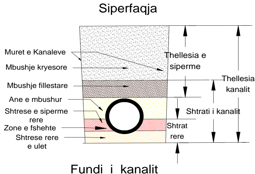
Figura 1 Kanali tipik i vendosjes se tubit dhe detajet e mbushjes
