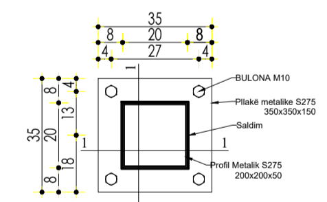
RAST I LIDHJA PROFILIT 200x200x5 MBI TRA PRERJA 1-1
