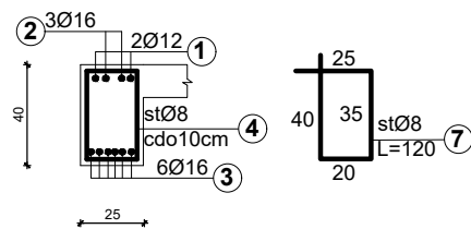
Prerja 1-1 e Tth-3 Shk 1:25
