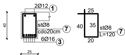
Prerja 2-2 e Tth-3 Shk 1:25
