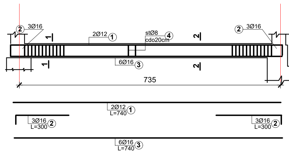
Prerja 1-1 e Tth-4 Shk 1:25
