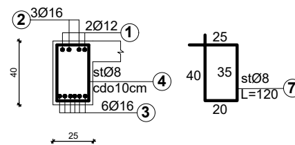
Prerja 1-1 e Tth-4 Shk 1:25
