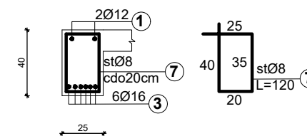
Prerja 1-1 e Tth-4 Shk 1:25
