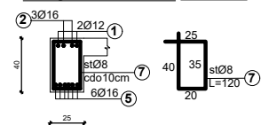
Prerja 1-1 e Tth-2 Shk 1:25
