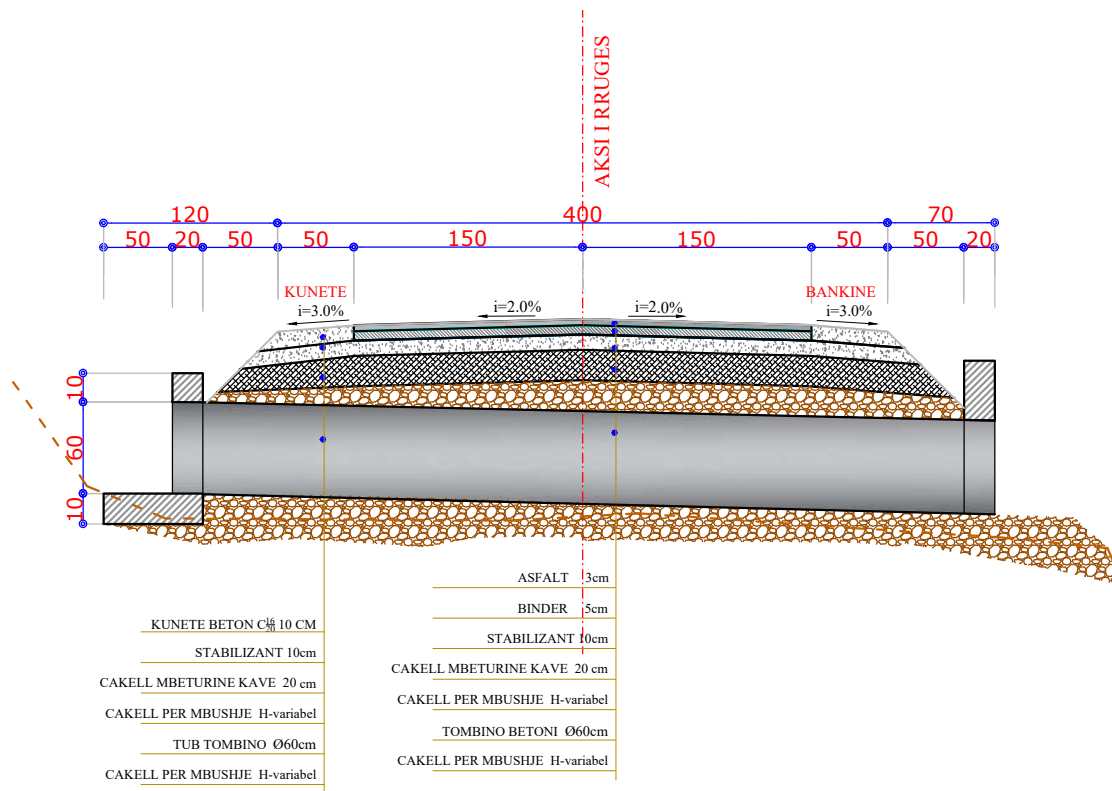
PROFIL TERTHOR TIP 4 (ME TOMBINO BETONI) SHK. 1:30
