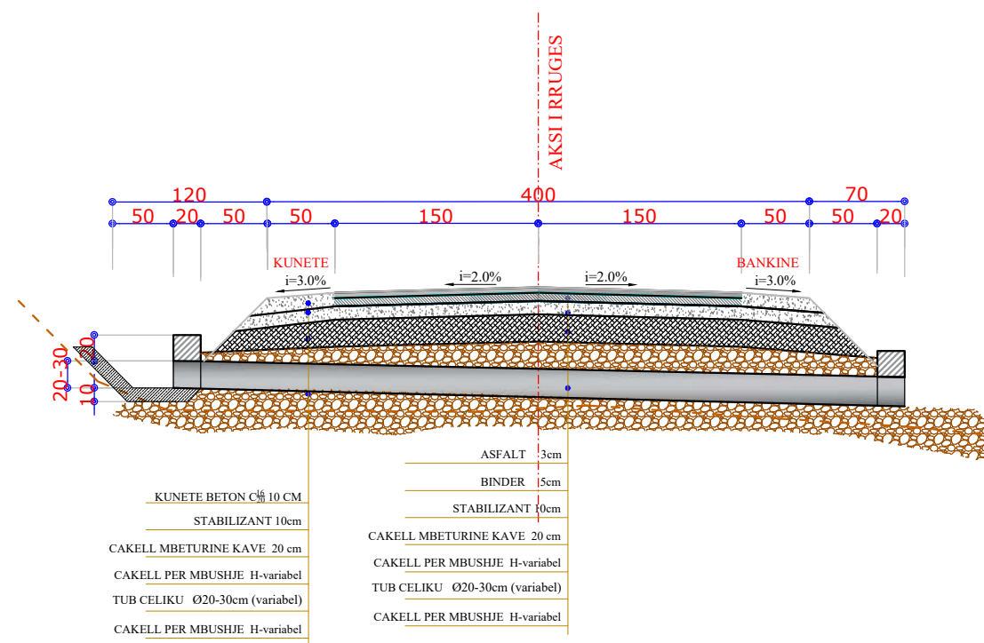
PROFIL TERTHOR TIP 5 (ME TUB CELIKU DHE KANAL KULLIMI) SHK. 1:30
