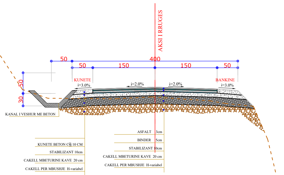
PROFIL TERTHOR TIP 3 (ME KANAL KULLIMI) SHK. 1:30
