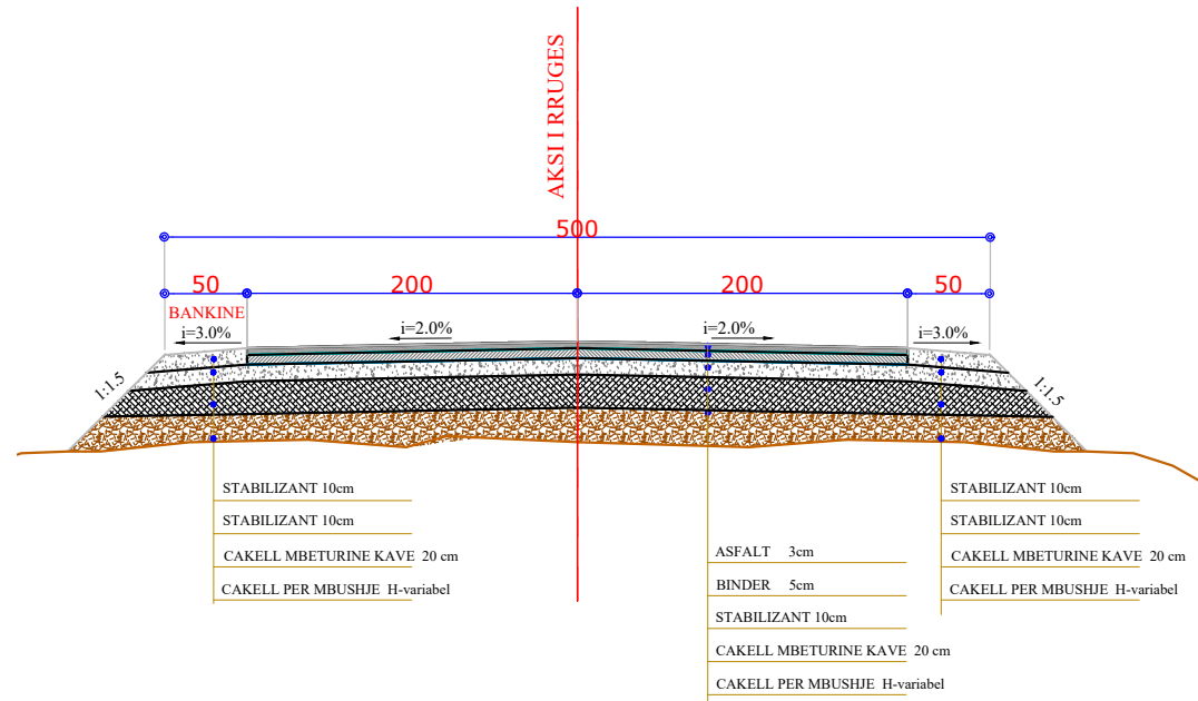
PROFIL TERTHOR TIP 1 (ME BANKINE) SHK. 1:30
