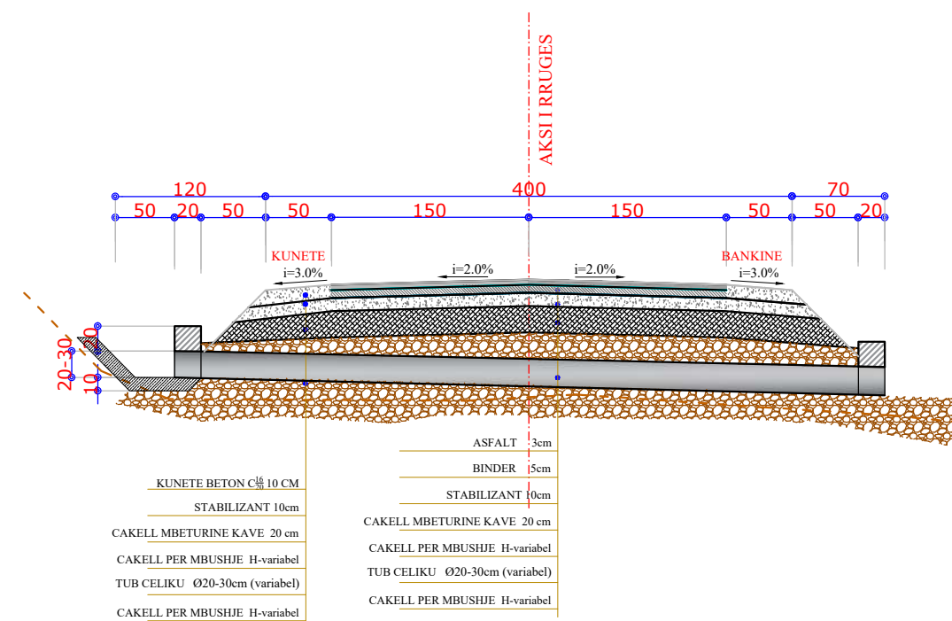
PROFIL TERTHOR TIP 5 (ME TUB CELIKU DHE KANAL KULLIMI) SHK. 1:30
