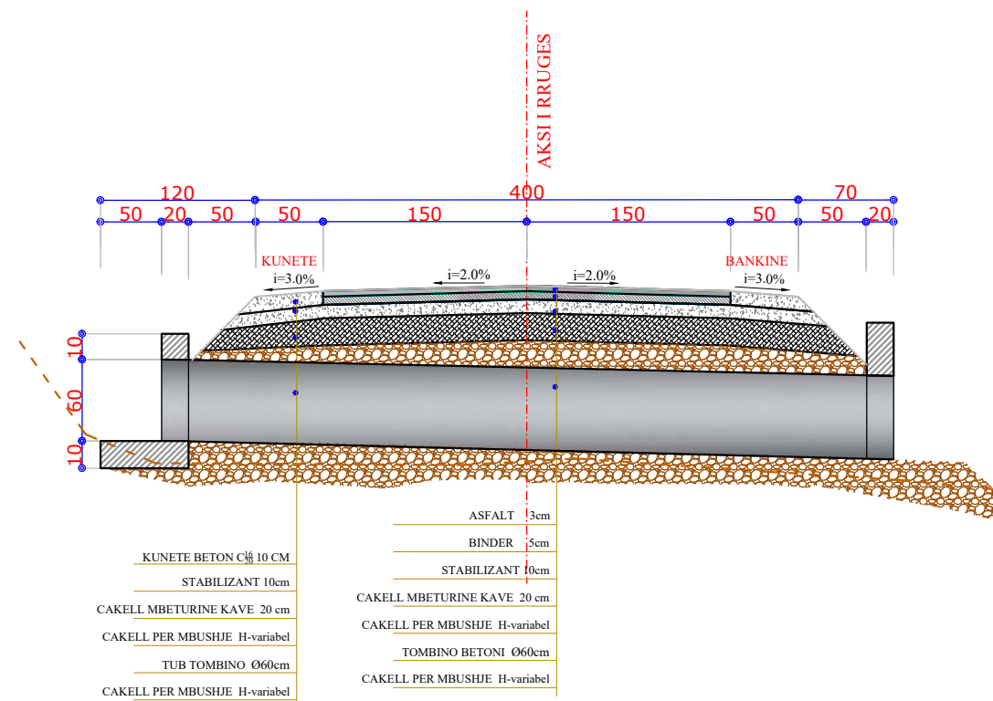
PROFIL TERTHOR TIP 4 (ME TOMBINO BETONI) SHK. 1:30
