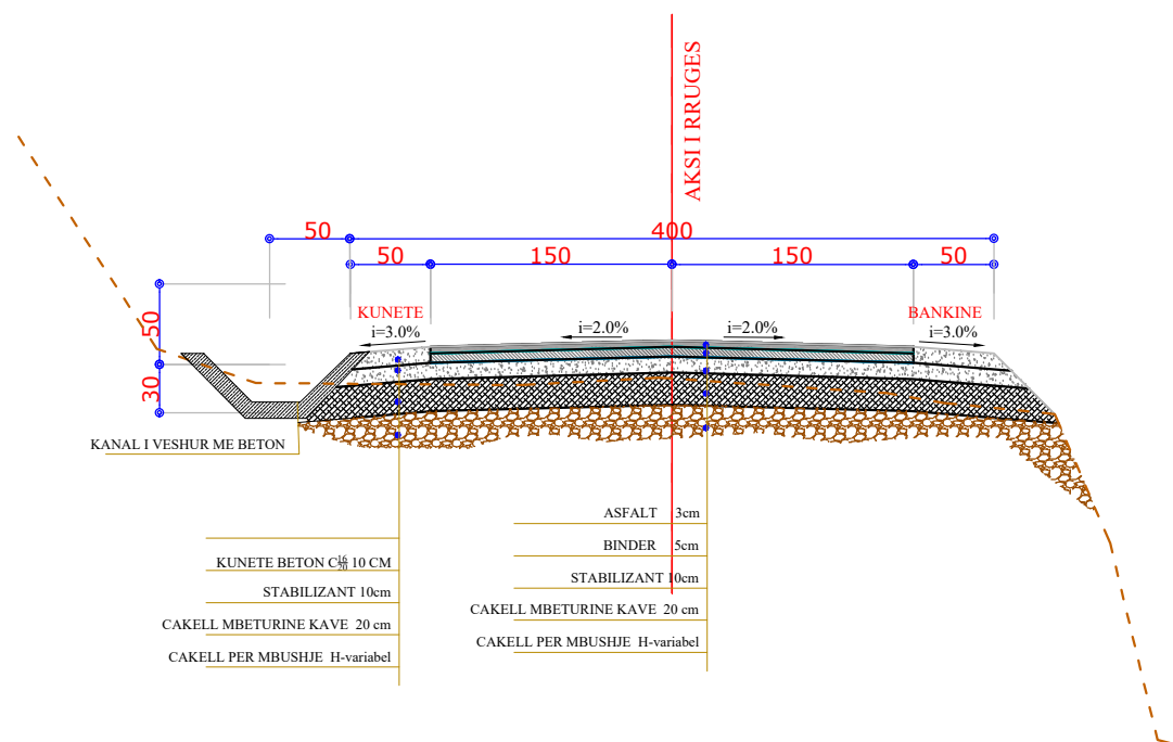
PROFIL TERTHOR TIP 3 (ME KANAL KULLIMI) SHK. 1:30
