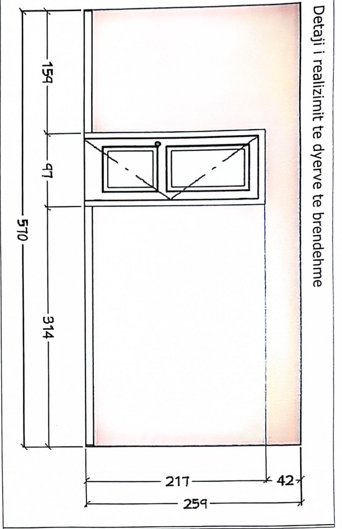
Detaji i realizimit te dritareve
