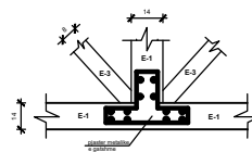
DETAJ D-2 SHK 1:20
