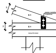
DETAJ D-3 SHK 1:20
