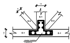
DETAJ D-2 SHK 1:20
