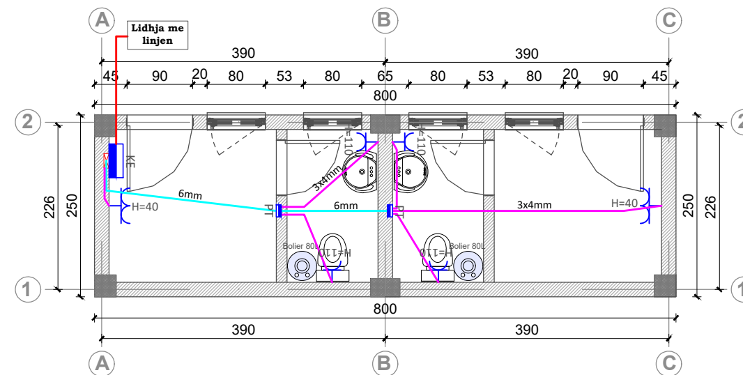
PLANIMETRIA E PRIZAVE/FUQISE
