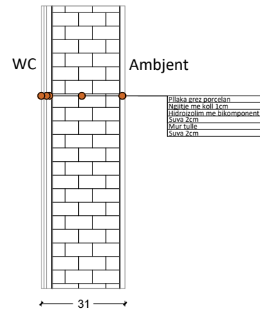
MUR I jashtem i tualetit LARTESIA E HIDROIZOLIMIT BIKOMPONENT 40CM
