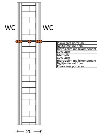
MUR I brendshem i tualetit/interior toilets wall LARTESIA E HIDROIZOLIMIT MR BIKOMPONENT 120CM
