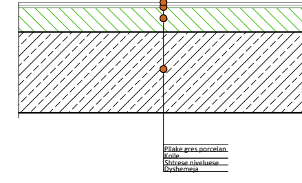
DETAJ DYSHEMEJE AMBIENTESH
