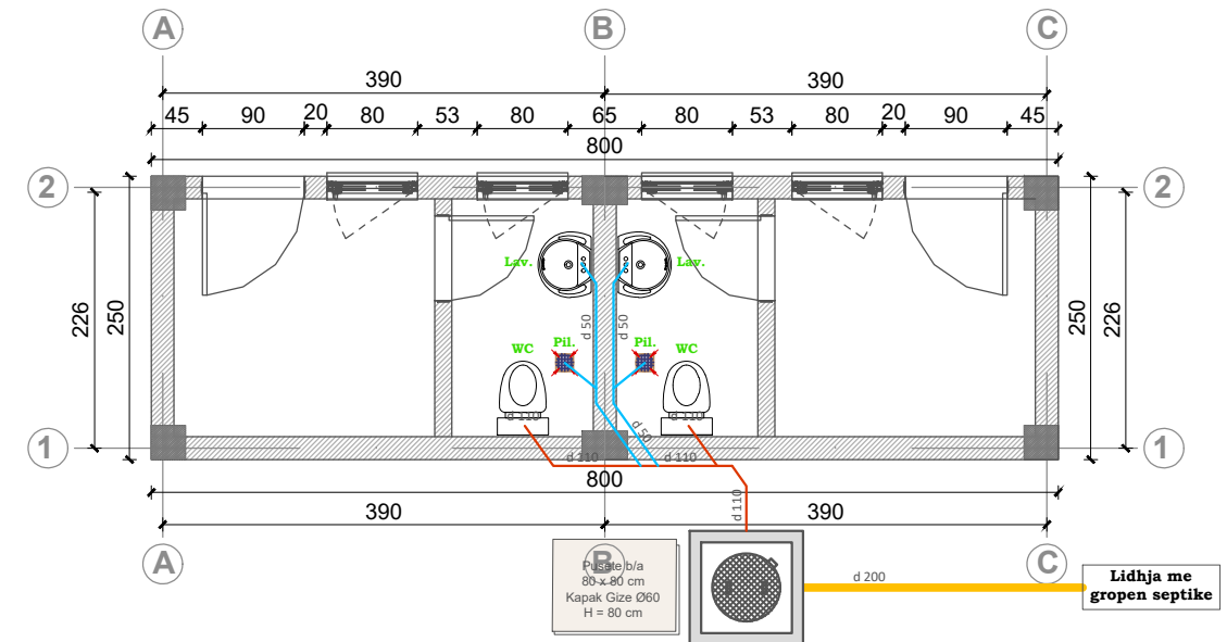
PLANIMETRIA E SHKARKIMEVE
