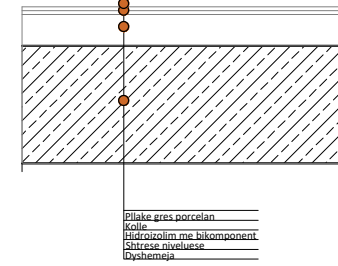
SHTRESAT E SHTRIMIT TE TUALETEVE
