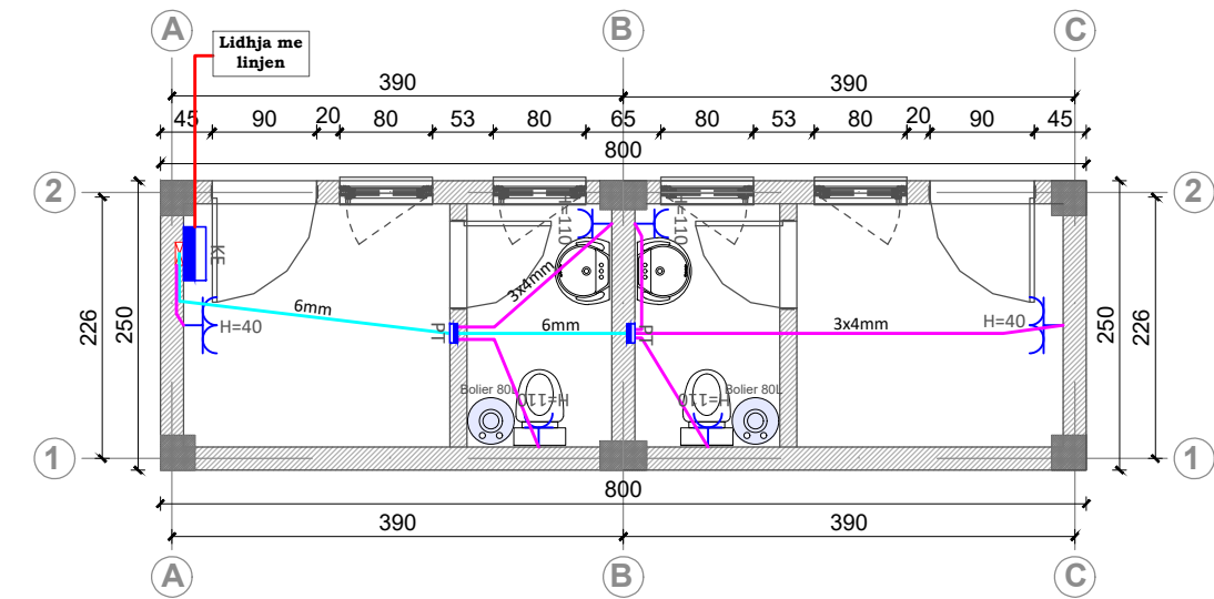
PLANIMETRIA E PRIZAVE/FUQISE
