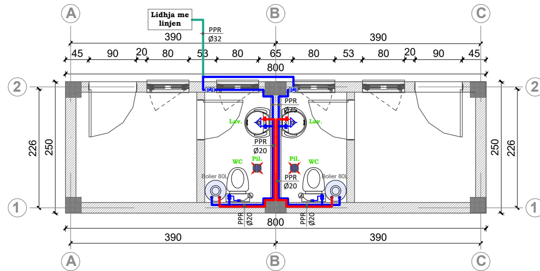
PLANIMETRIA E F.U
