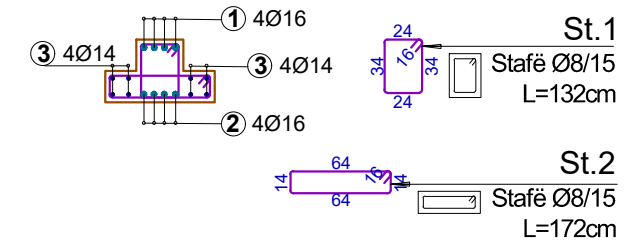
Prerja 1-1
