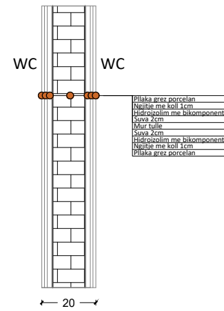
MUR I brendshem i tualettit/interior toilets wall LARTESIA E HIDROIZOLIMIT MR BIKOMPONENT 120CM
