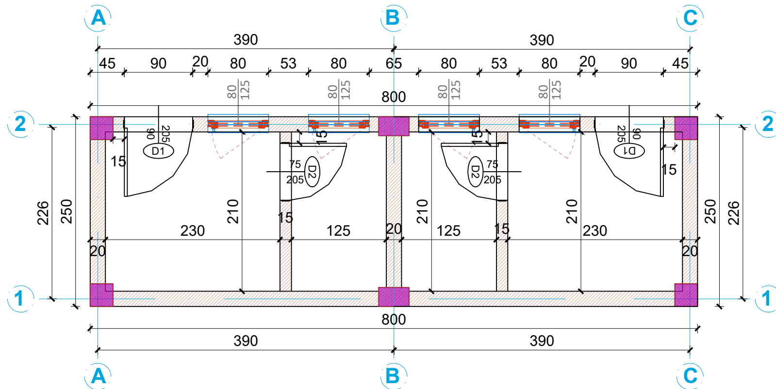
PLANIMETRIA TEKNIKE
