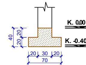
Prerja tip
