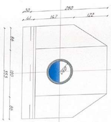
SEKSIONI TERTHOR I KANALIT MATERIAL I SHKRIFJET RERE 10CM
