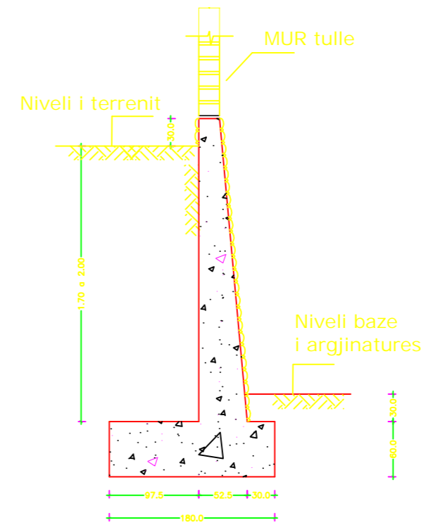
Seksio i nje muri dhembajtes ne afersi te argjinatures
