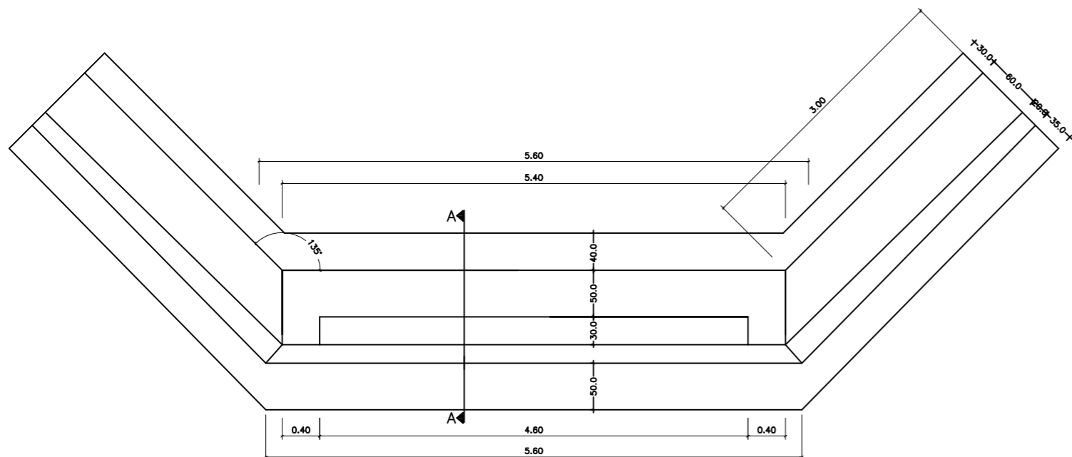
PLANIMETRI Shkalla 1-50
