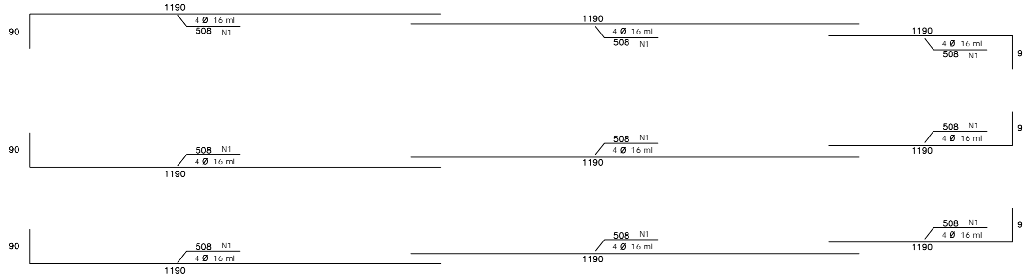
Hekur periodik anesor per lidhjen e trarit T-1
