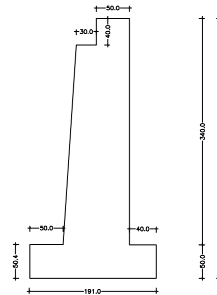
PRERJA A-A Shkalla 1-50
