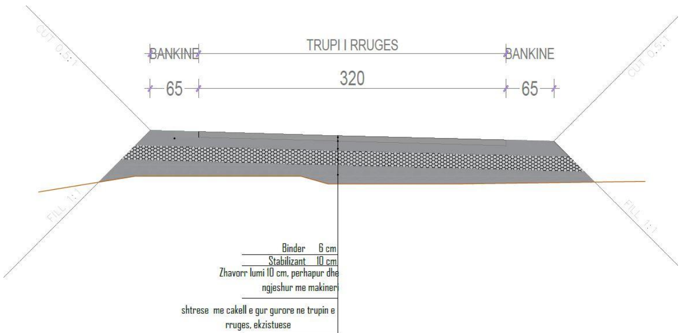
Profilu tip 1 ka trupin e rrugës me gjerësi 3.2 m, 2 bankina me gjerësi 0.65 m në secilën anë .
