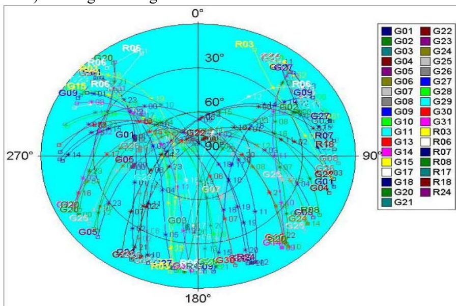
Diagrama e dukshmërisë satelitore Vlerat DOP për GPS dhe GLN
