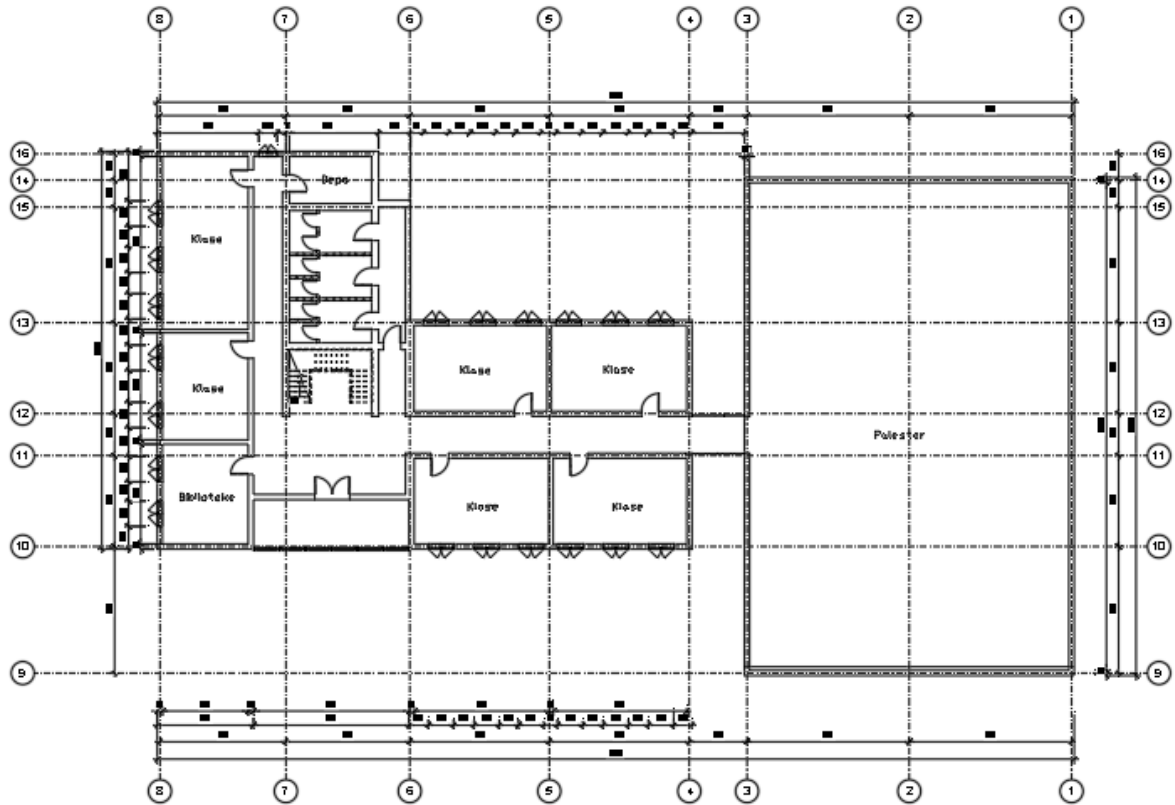
Planimetria e katit perdhe
