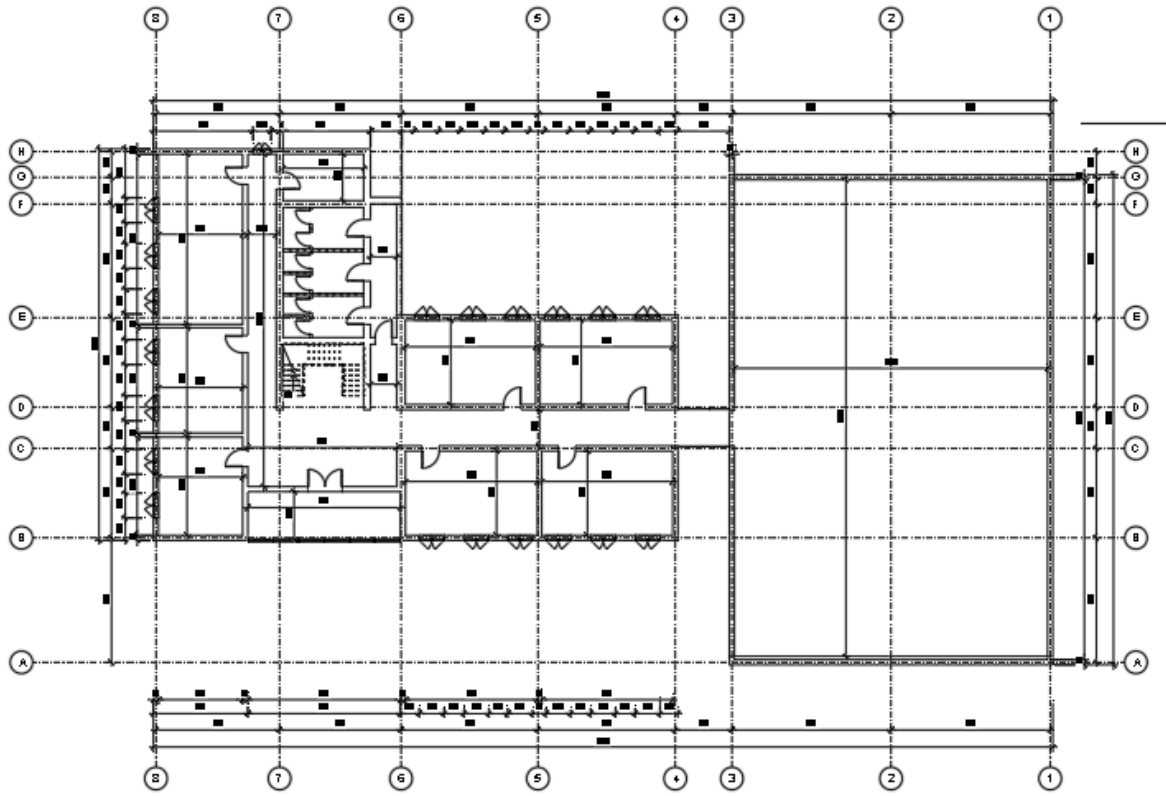
Planimetria e katit te I-re
