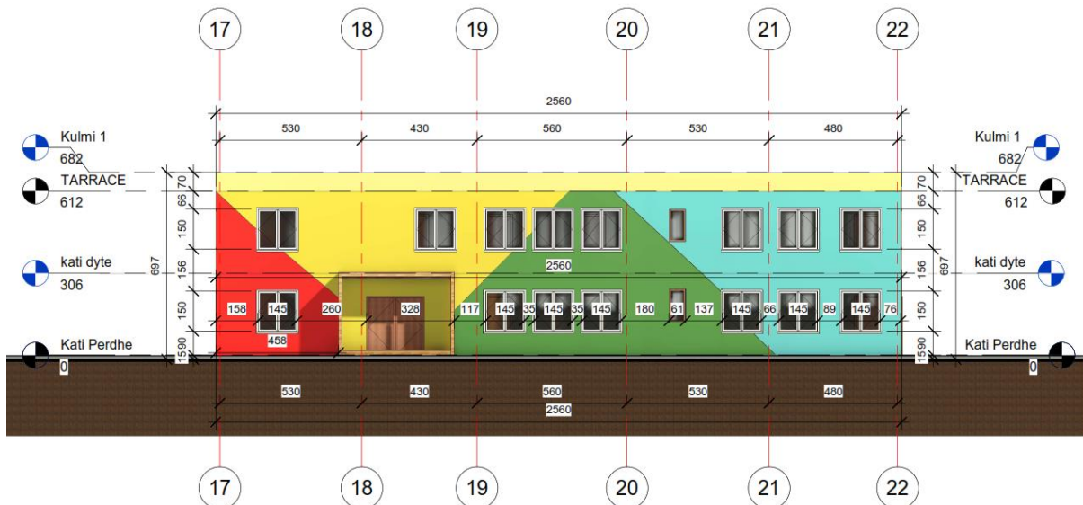
Fasada Veri Perendimore
