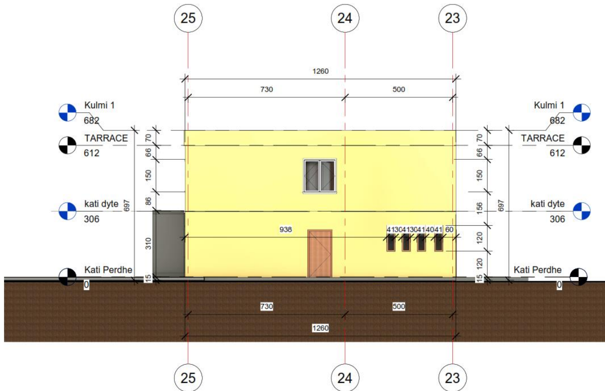
Fasada Jug Perendimore
