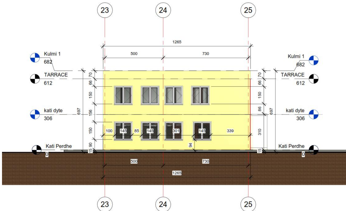
Fasada Veri Lindore
