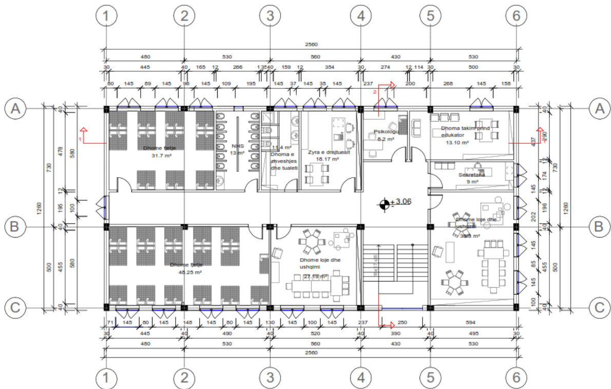
Planimetria e kopshit Kati i Pare
