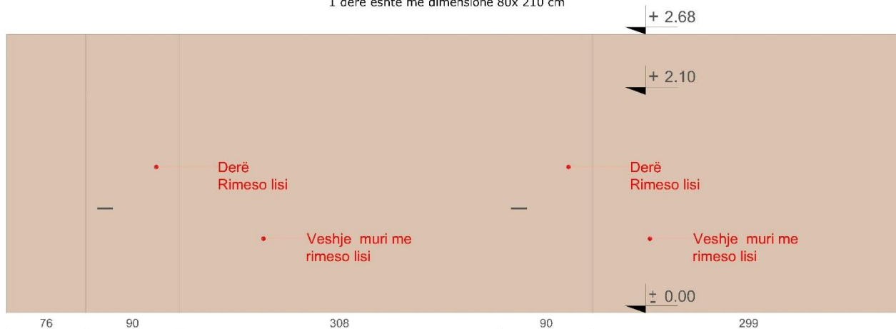
Pamja A-A
